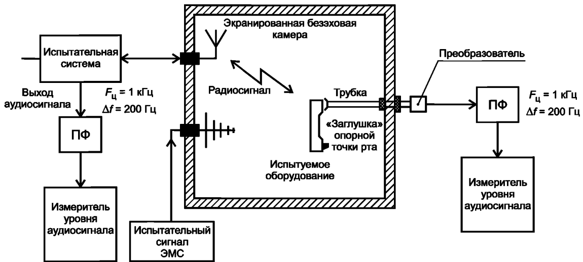
Рисунок 2 — Схема прохождения сигнала при испытаниях портативного оборудования
