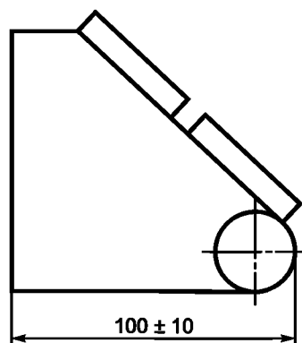
Рисунок В.1 — Специальное размещение горизонтального поста управления в кабине (вид сбоку)
