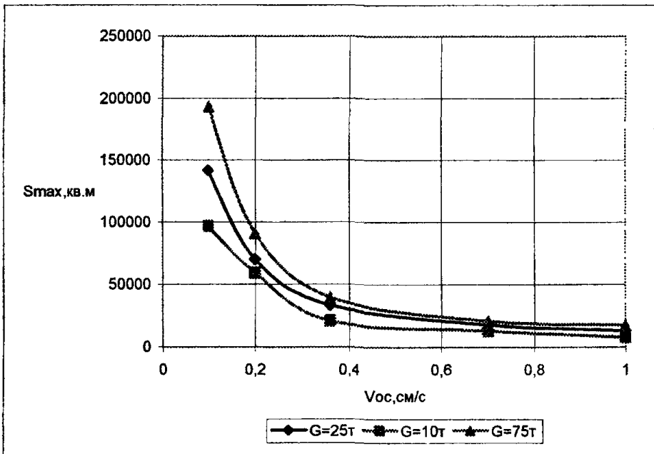
Рисунок 21 - Наибольшие площади S_{max} зон мутности на поверхности для ПДК=0,75мг/л (а) и для ПДК=0,25мг/л (б) при дампинге из трюма землесоса
