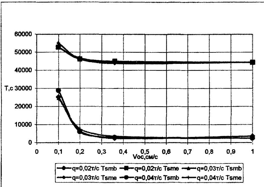
Рисунок 12 - Время T_{smb} достижения зонами мутности наибольших размеров на дне и момент T_{sme} начала их уменьшения для PDK=0,75 mg/l (а) и для PDK=0,25 mg/l (б) при дноуглублении черпаковыми земснарядами
