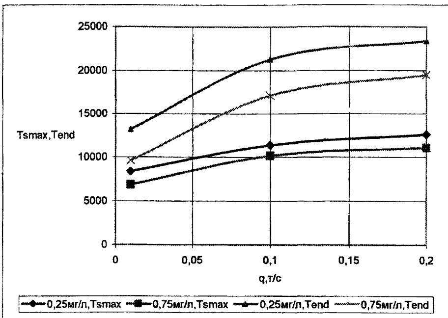
Рисунок 4 - Наибольшие площади зон мутности S_{max} на глубине d/2 для ПДК=0,75 мг/л и для ПДК=0,25 мг/л (а); моменты T_{max} достижения зон мутности наибольших размеров и моменты T_{end} их существования при дноуглублении землесосами V_{oc}=0,01 см/с (б)
