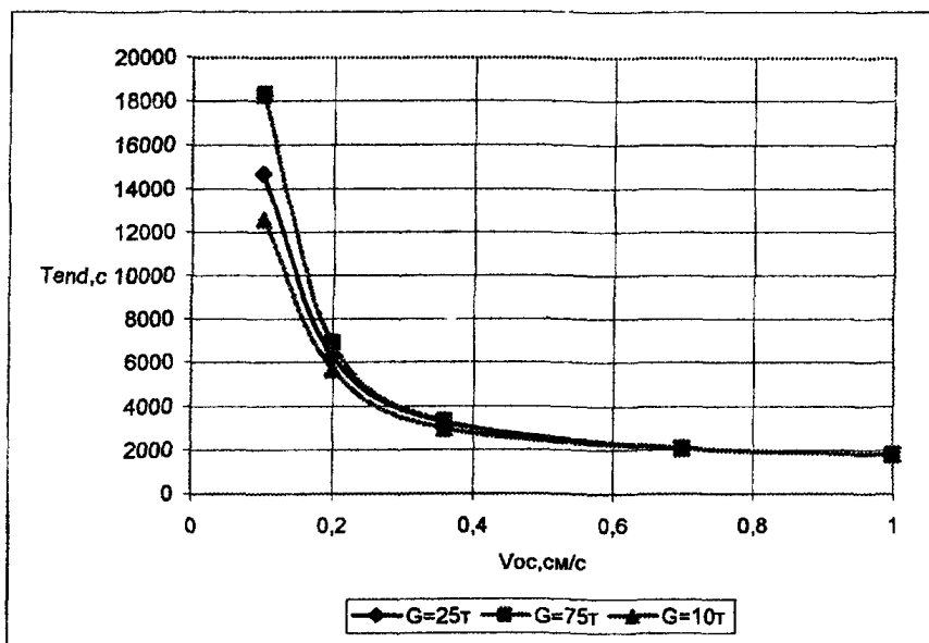
Рисунок 23 - Время T_{end} существования зон мутности на поверхности для ПДК=0,75мг/л (а) и для ПДК=0,25мг/л (б) при дамплинге из трюма землесоса
