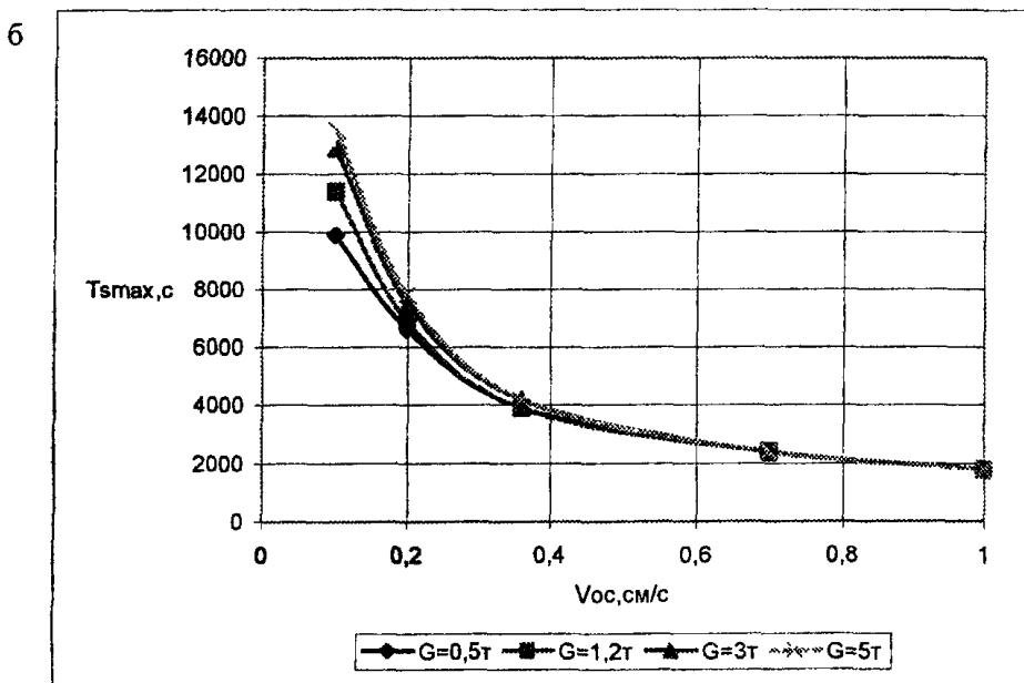
Рисунок 19 - Время T_{max} образования на глубине d/2 зон мутности наибольших размеров для ПДК=0,75мг/л (а) и ПДК=0,25мг/л (б) при дампинге из шаланд
