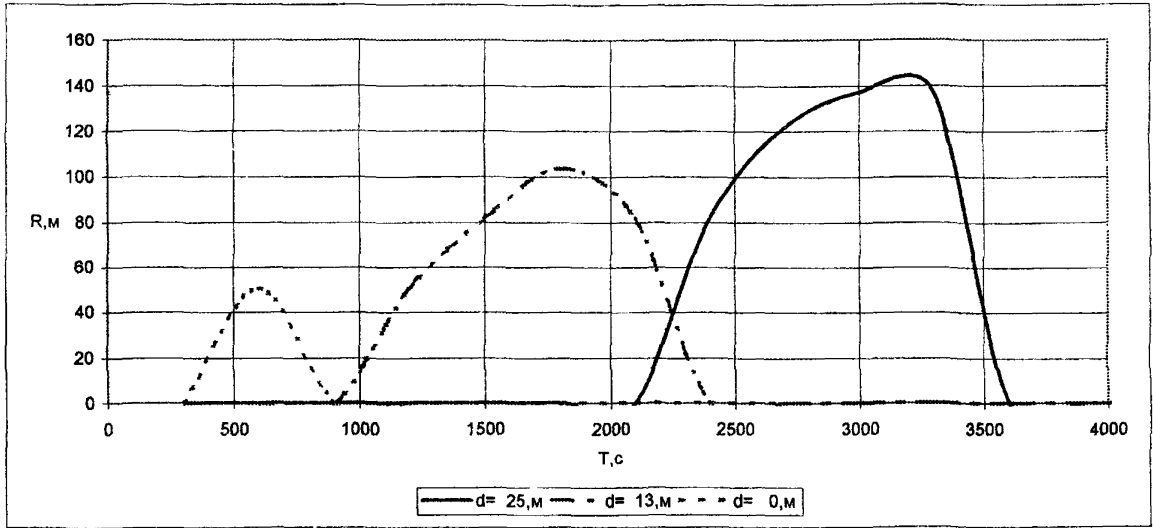
Рисунок Е.4 - Зависимость радиусов зон мутности R_1 на трех горизонтах от времени T , прошедшего с момента сброса при глубине 25 м
