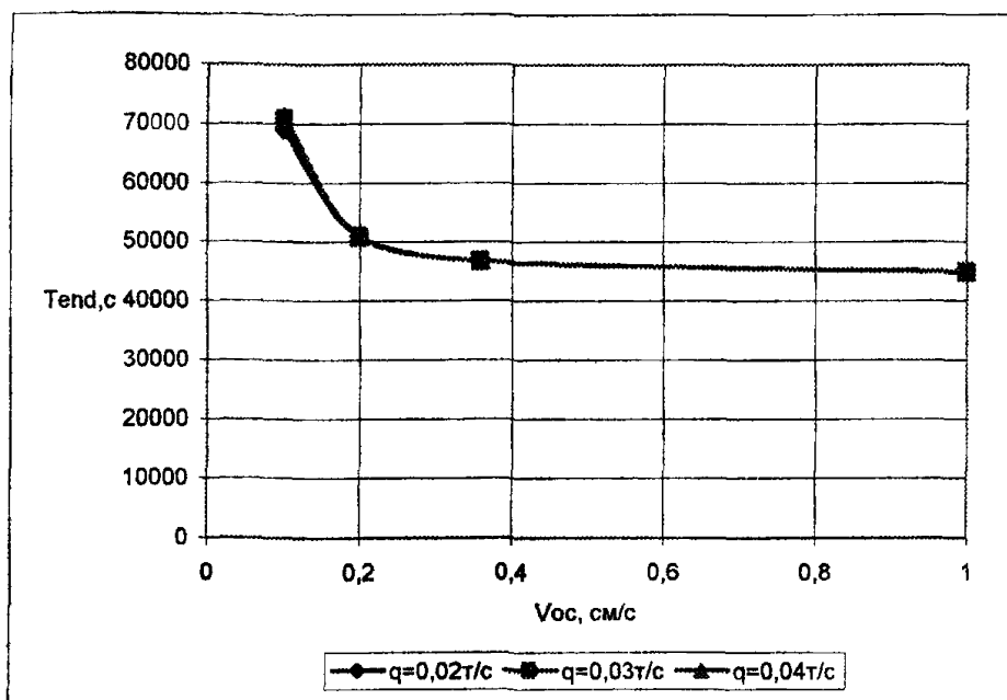
Рисунок 13- Время существования T_{end} зон мутности на дне для ПДК=0,75мг/л (а) и для ПДК=0,25мг/л (б) при дноуглублении черпаковыми земснарядами
