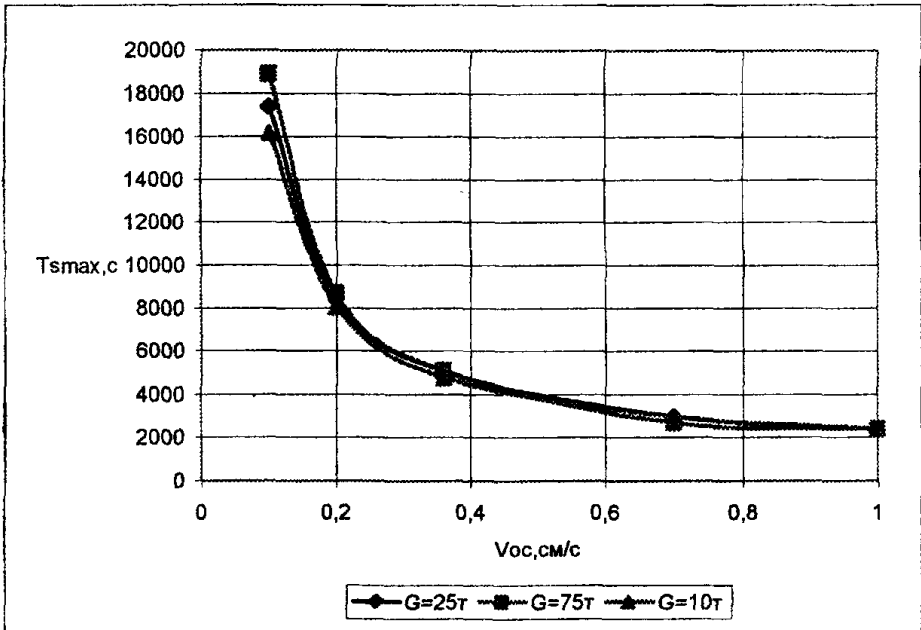
Рисунок 25 - Время T_{\text{smax}} образования на глубине d/2 пятна взвеси наибольших размеров для ПДК=0,75мг/л (а) и ПДК=0,25мг/л (б) при дампинге из трома землесоса
