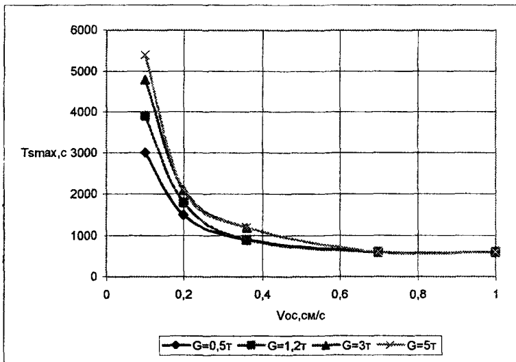
Рисунок 16 - Время T_{smax} образования на поверхности зон мутности наибольших размеров для ПДК=0,75мг/л (а) и ПДК=0,25мг/л (б) при дамплинге из шаланд
