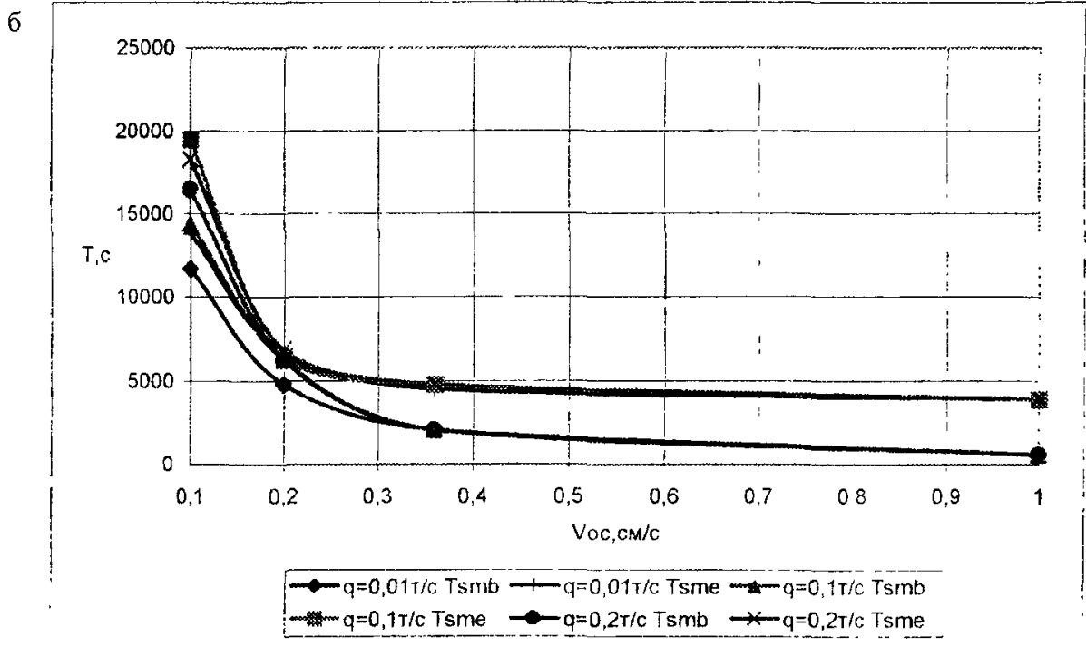
Рисунок 2 - Время T_{smb} достижения зонами мутности на дне наибольших размеров и начала их уменьшения T_{sme} для ПДК = 0,75 мг/л (а) и для ПДК=0,25мг/л при дноуглублении землесосами
