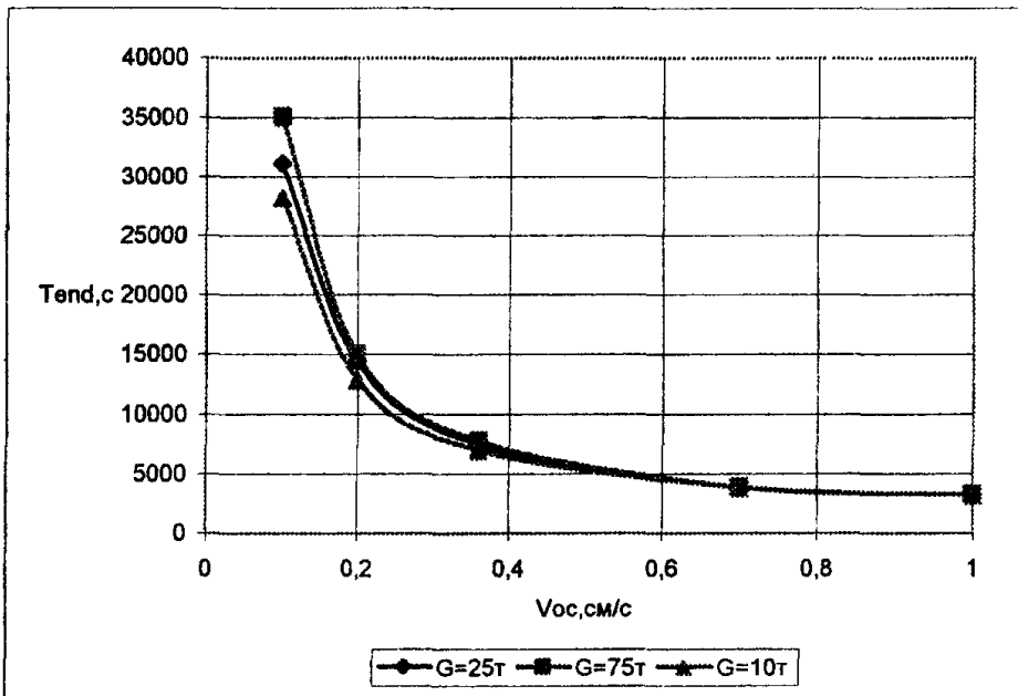
Рисунок 26 - Время T_{end} существования зон мутности на глубине d/2 для ПДК=0,75мг/л (а) и для ПДК=0,25мг/л (б) при дампинге из трюма землесоса
