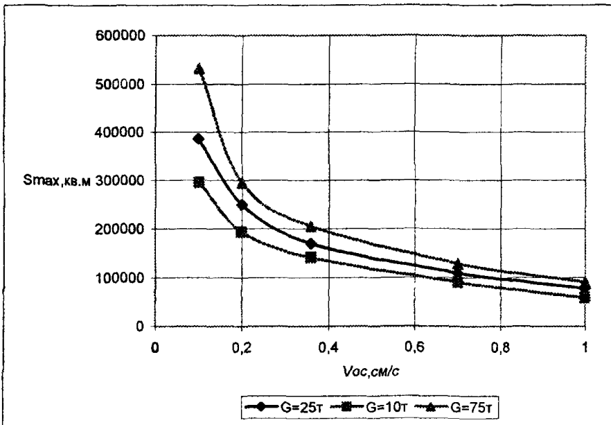
Рисунок 24 - Наибольшие площади S_{max} зон мутности на глубине d/2 для ПДК=0,75 мг/л (а) и для ПДК=0,25 мг/л (б) при дампинге из трюма землесоса
