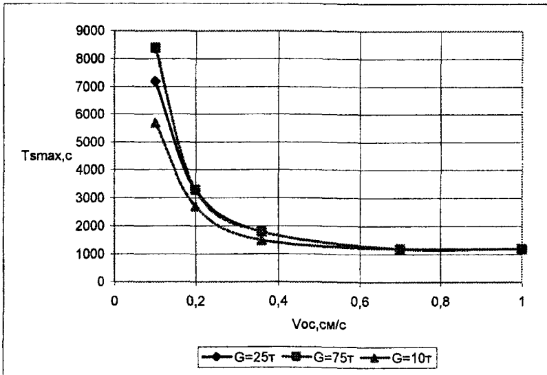
Рисунок 22 - Время T_{max} образования на поверхности зон мутности наибольших размеров для ПДК=0,75мг/л (а) и ПДК=0,25мг/л (б) дампинге из гряда землесоса
