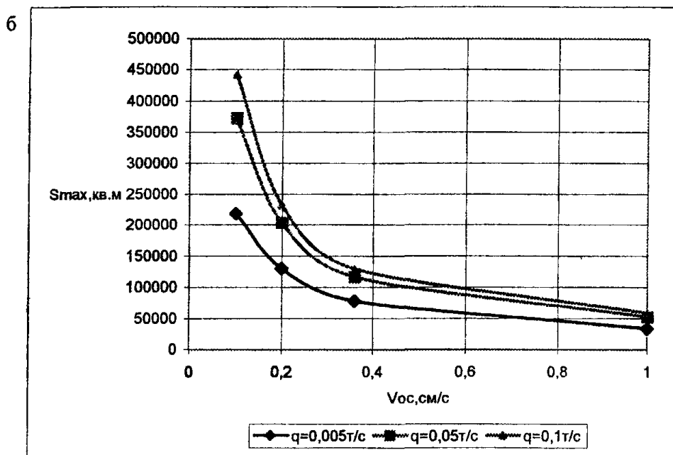
Рисунок 8 - Наибольшие площади S_{max} зон мутности на глубине d/2 для ПДК=0,75 мг/л (а) и для ПДК=0,25 мг/л (б) при сливе из труба землесоса во время его работы
