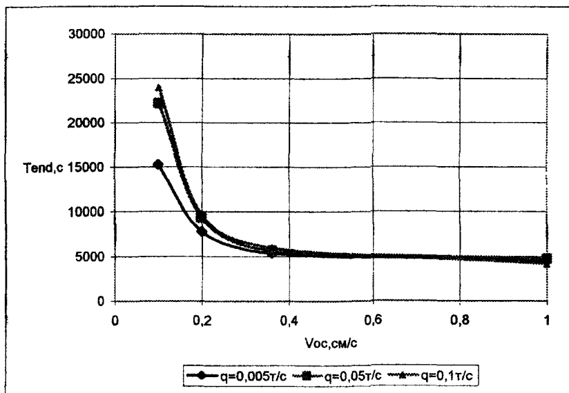
Рисунок 7 - Время Tенд существования на поверхности зон мутности для ПДК=0,75мг/л (а) и для ПДК=0,25мг/л(б) при сливе из трюма землесоса во время его работы
