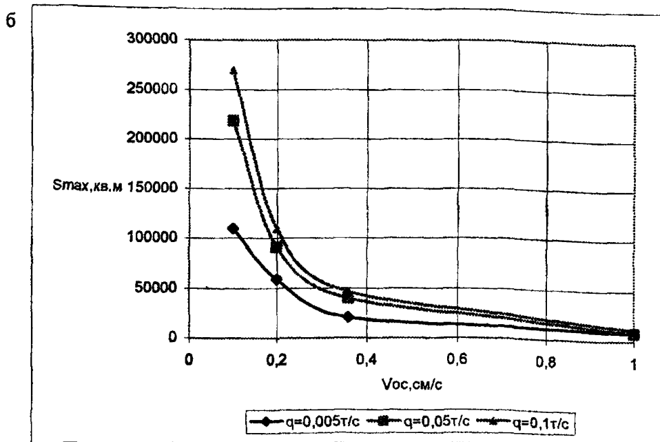
Рисунок 5 - Наибольшие площади S_{max} зон мутности на поверхности для ПДК=0,75мг/л (а) и для ПДК=0,25 мг/л (б) при сливе из трюма землесоса во время его работы
