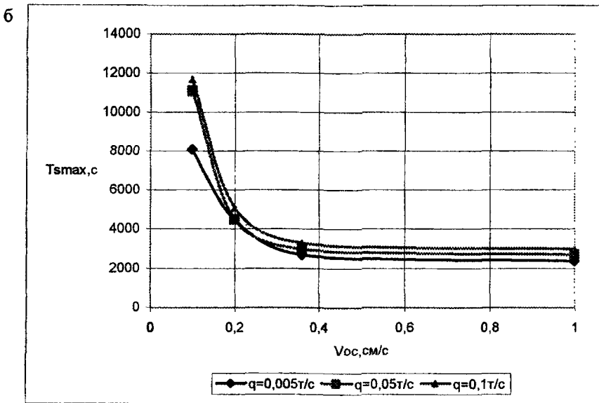
Рисунок 6 - Время T_{smax} образования на поверхности зон мутности наибольших размеров для ПДК=0,75мг/л (а) и ПДК=0,25мг/л(б) при сливе из трюма землесоса во время его работы
