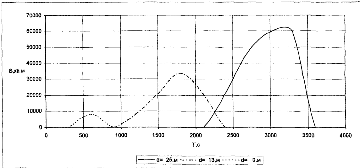
Рисунок Е.3 - Зависимость площадей зон мутности S_1 на трех горизонтах от времени T , прошедшего с момента сброса при глубине 25 м
