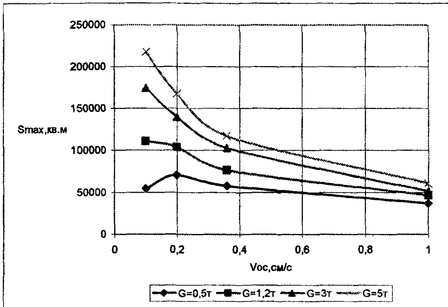
Рисунок 18 - Наибольшие площади S_{max} зон мутности на глубине d/2 для ПДК=0,75 мг/л (а) и для ПДК=0,25 мг/л (б) при дамплинге из шаланд
