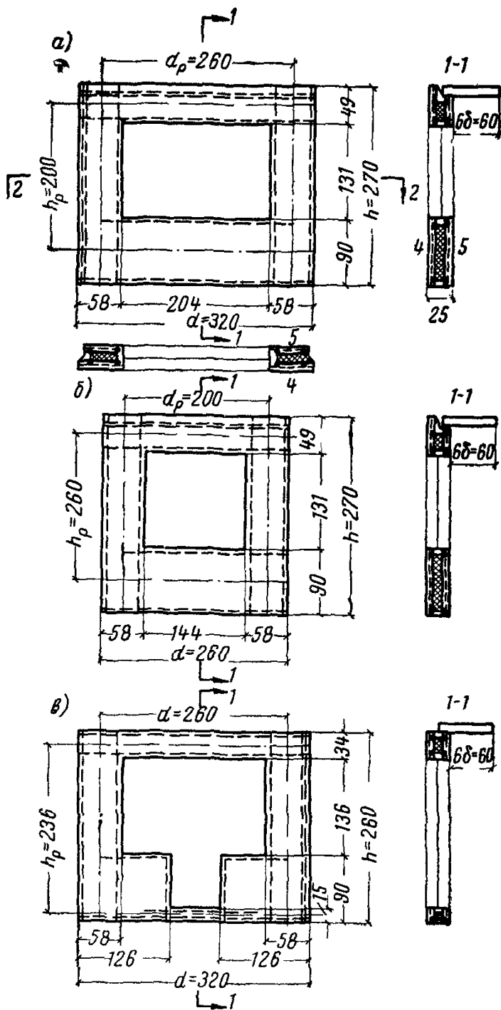
Рис. V.5. Схемы наружных стеновых панелей
