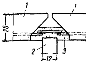
Рис. V.4. Стык между панелями наружной продольной стены
