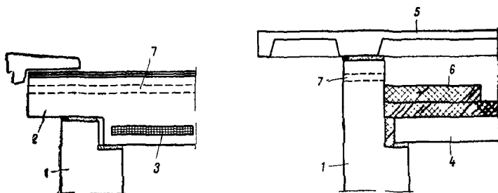
Рис. 22. Теплоизоляция горизонтального стыка наружных стен с панелями совмещенных и отдельных крыш
