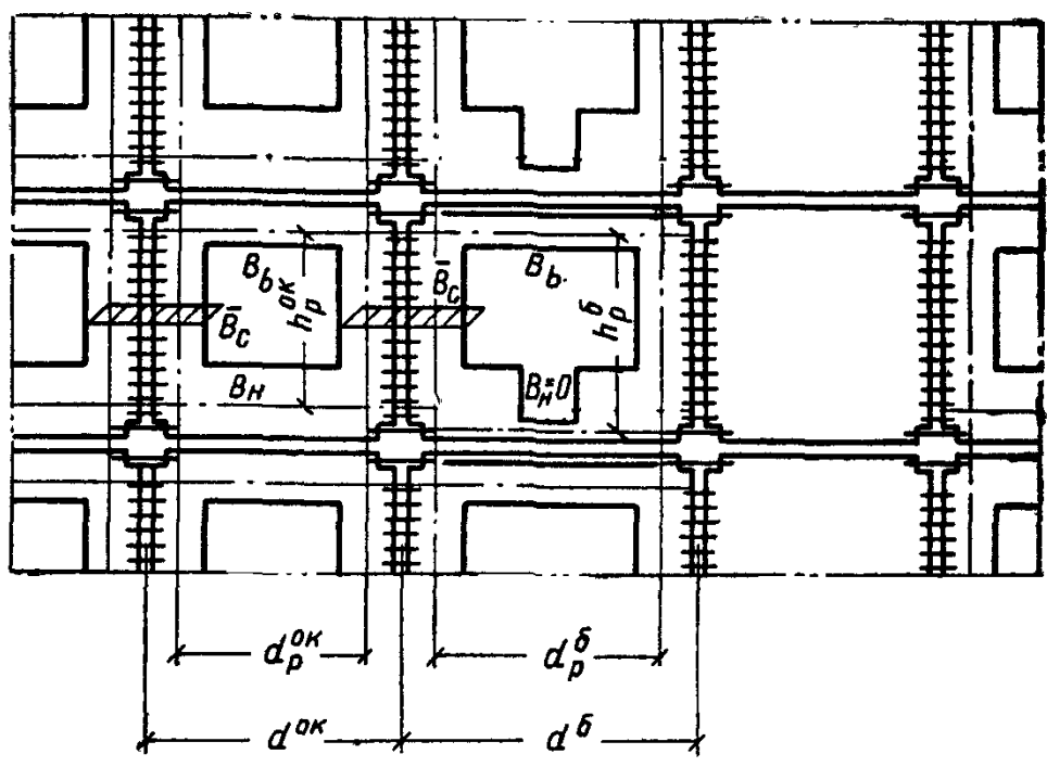
Рис. IV.5. К определению жесткой характеристики панели при перекосе
