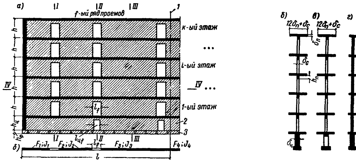
Рис. IV.3. Схема внутренней продольной стены
