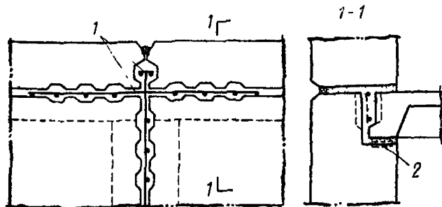
Рис. 14. Связь панелей стен и перекрытий замоноличиваемыми арматурными каркасами
