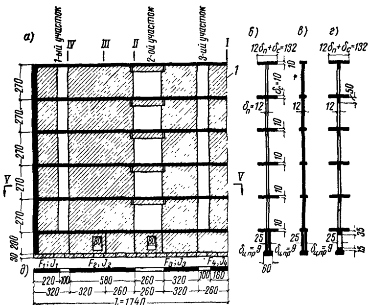
Рис. V.7. Схема внутренней продольной стены
