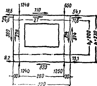
Рис. V.15. Схема нагрузок на наружную стеновую панель 1-го этажа 2-го столба
