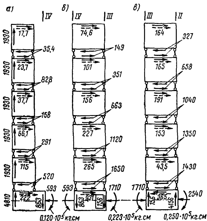
Рис. V.11. Схема усилий во внутренней продольной стене а — первый столбец; б — второй столбец; в — третий столбец
