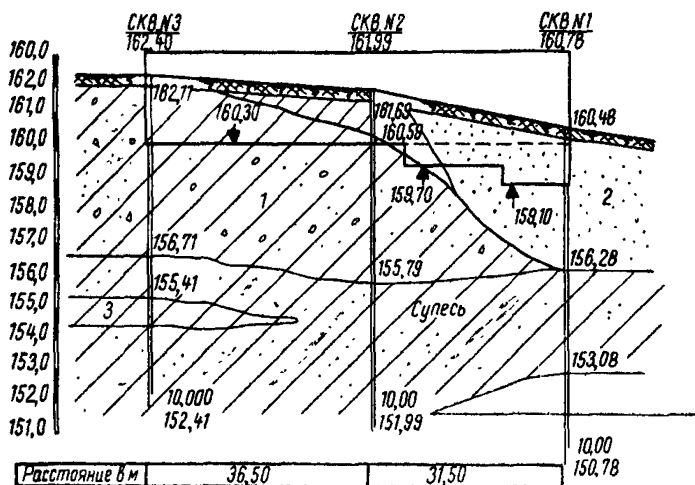
Рис. V.16. Геологический профиль
