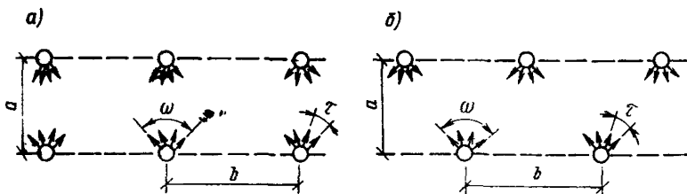
Рис. 1. Схемы расположения осветительных приборов
