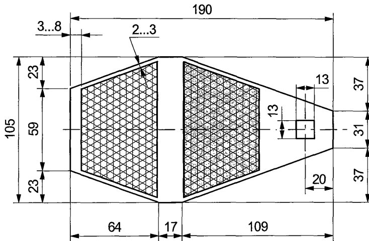
Развертка
