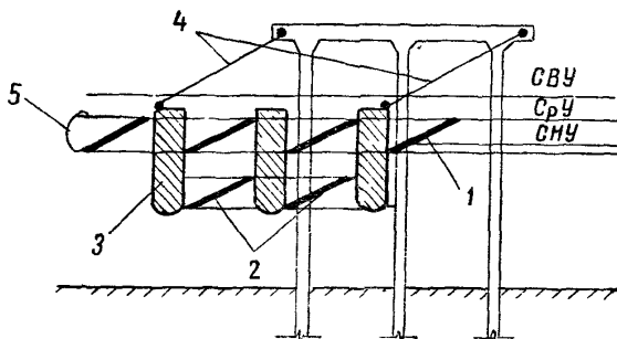
Рис. 13. Схема волнолома с гасителем, имеющим плоскопоступательную подвижность
