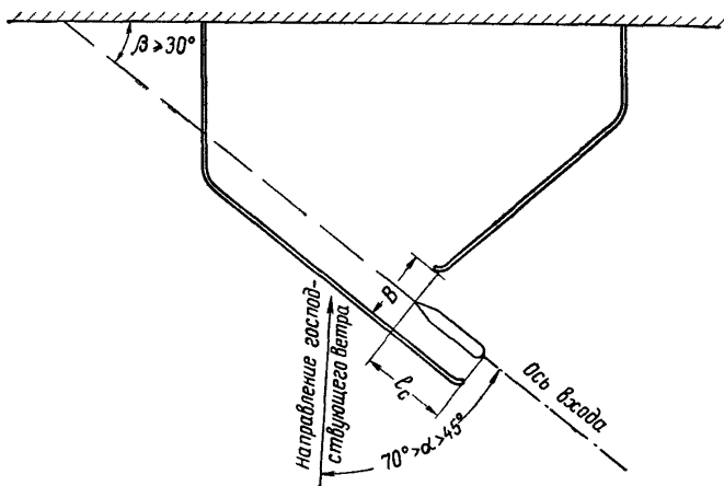
Рис 2 Схема к определению ширины входа в порт
