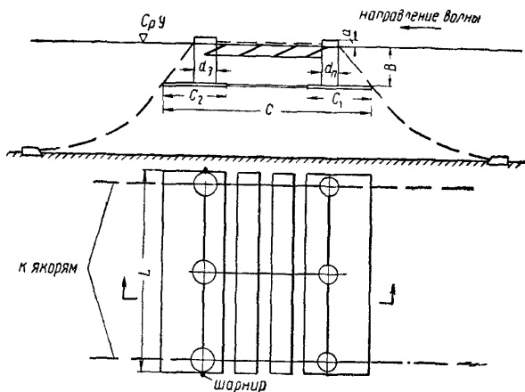
Рис 15 Схема плавучего волнолома
