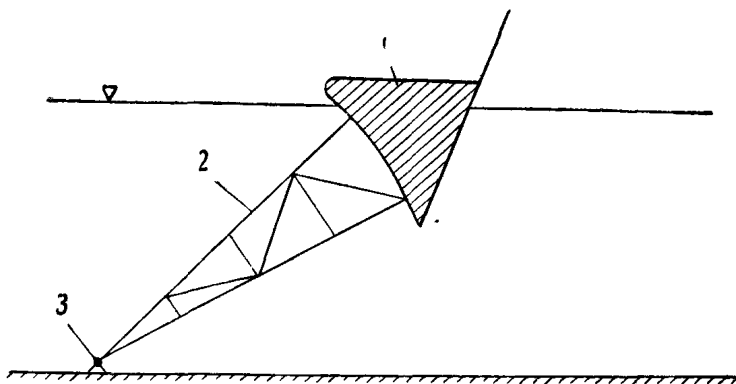
Рис 14 Схема качающегося волнолома 1 — плавучий корпус, 2 — ферма, 3 — шарнир
