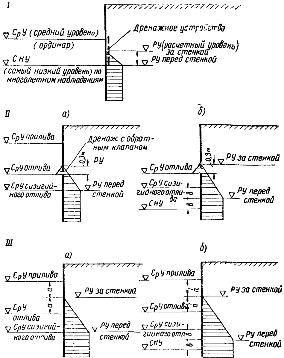
Рис 5. Расчетные давления воды на стенки свайных двухрядных конструкций
