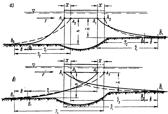
Рис 16. Несимметричные системы заякорения
