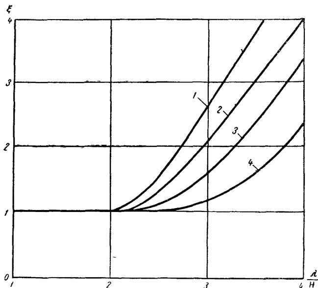
Рис 11 График для определения коэффициента \xi
