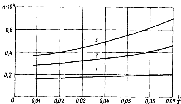
Рис 10 График для определения коэффициента k 1 — при k_r = 0,25 2 — при k_r = 0,50 . 3 — при k_r = 0,75
