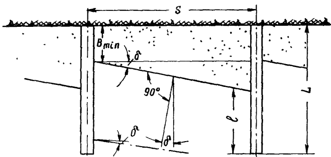
Рис 18 Схема для определения расчетной длины бун
