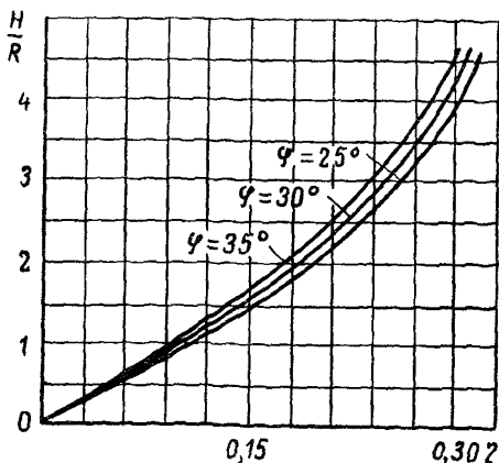
Рис. 6. График для определения коэффициента \eta
