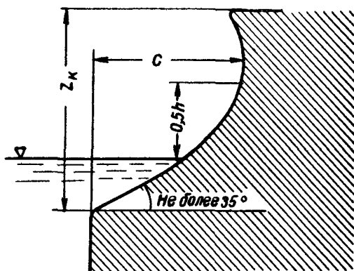
Рис 17. Волнозащитная стена с волноотражательным козырьком
