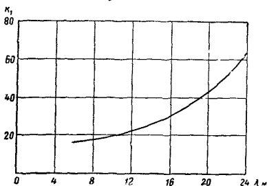
Рис. 12. График для определения коэффициента \kappa_1
