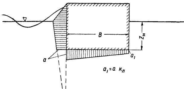
Рис 21 Схема для определения взвешивающего давления на экран ящичного типа
