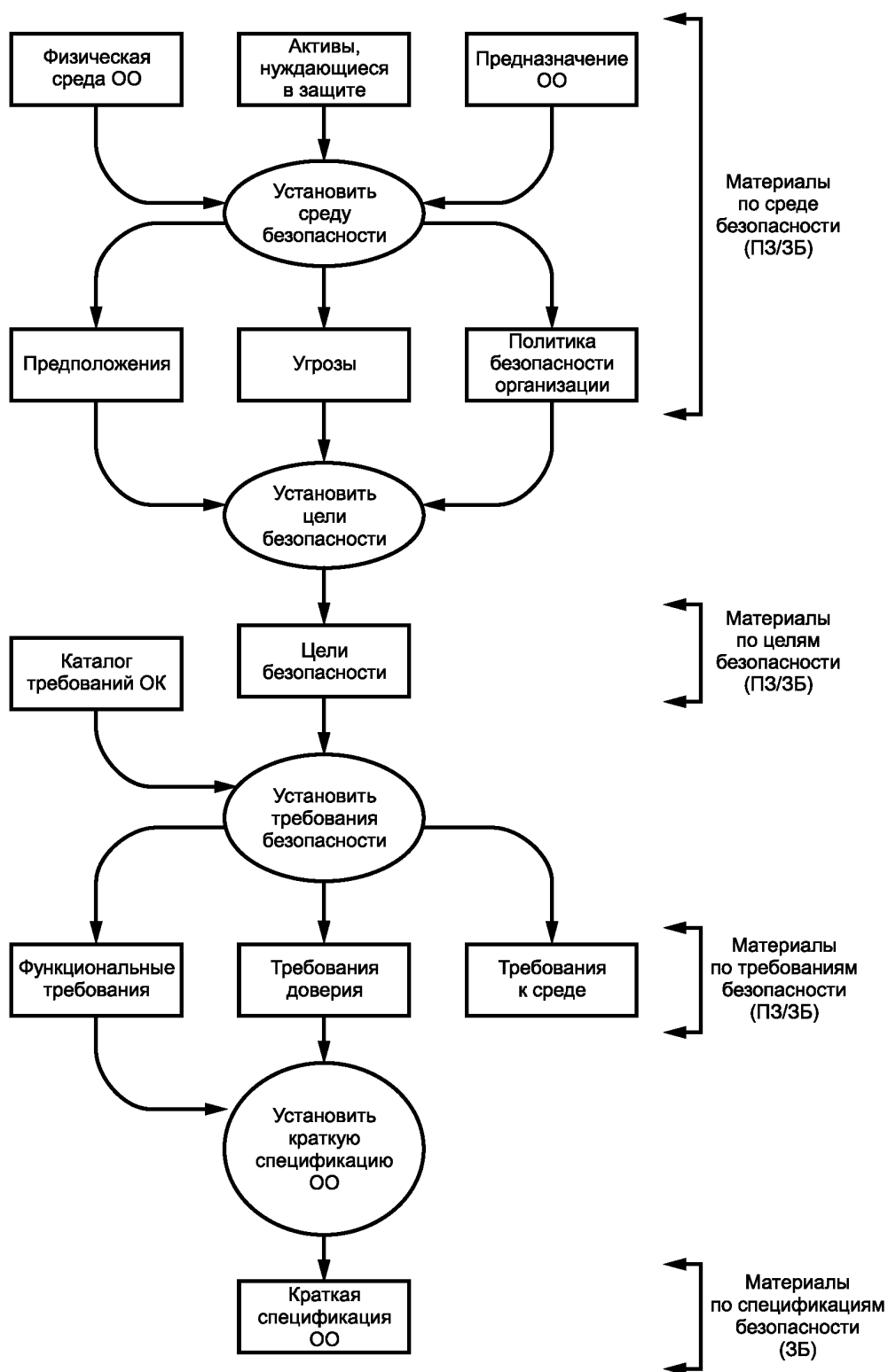
Рисунок 6 — Последовательное формирование требований и спецификаций
