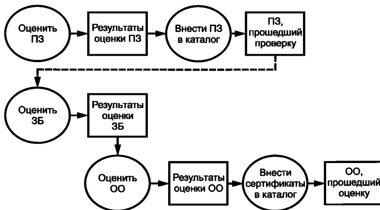
Рисунок 9 — Результаты оценки
