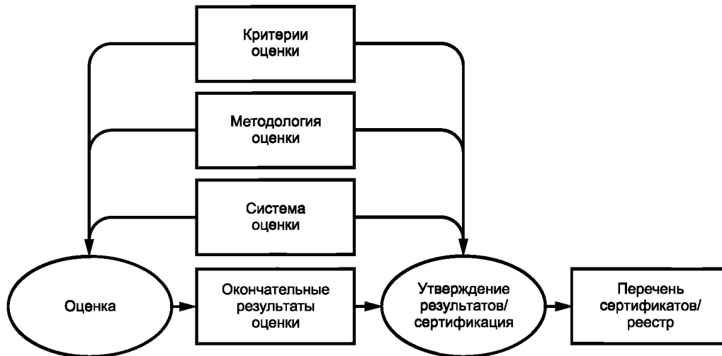
Рисунок 1 — Контекст оценки
