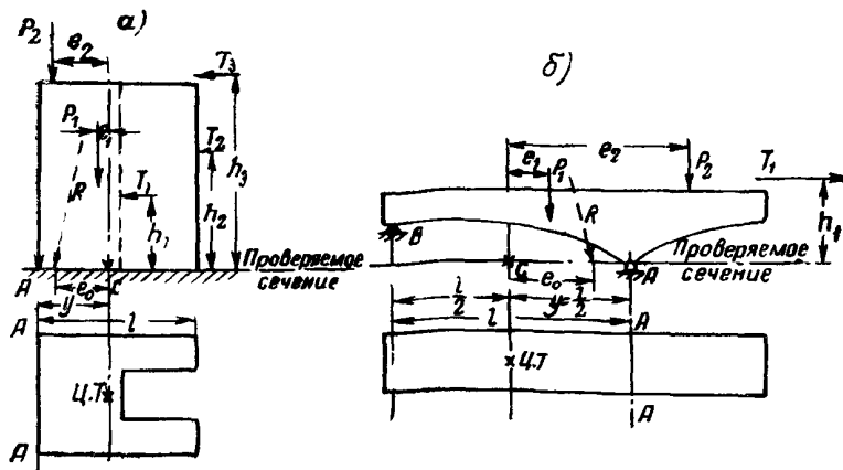
Рис. 1. Схемы к расчету на устойчивость против опрокидывания при опирании
