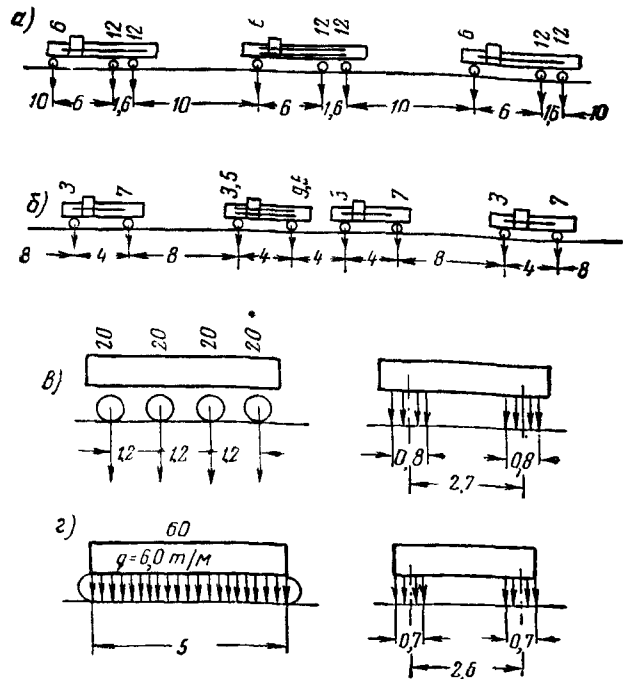
Давления в тоннах Расстояния в метрах
