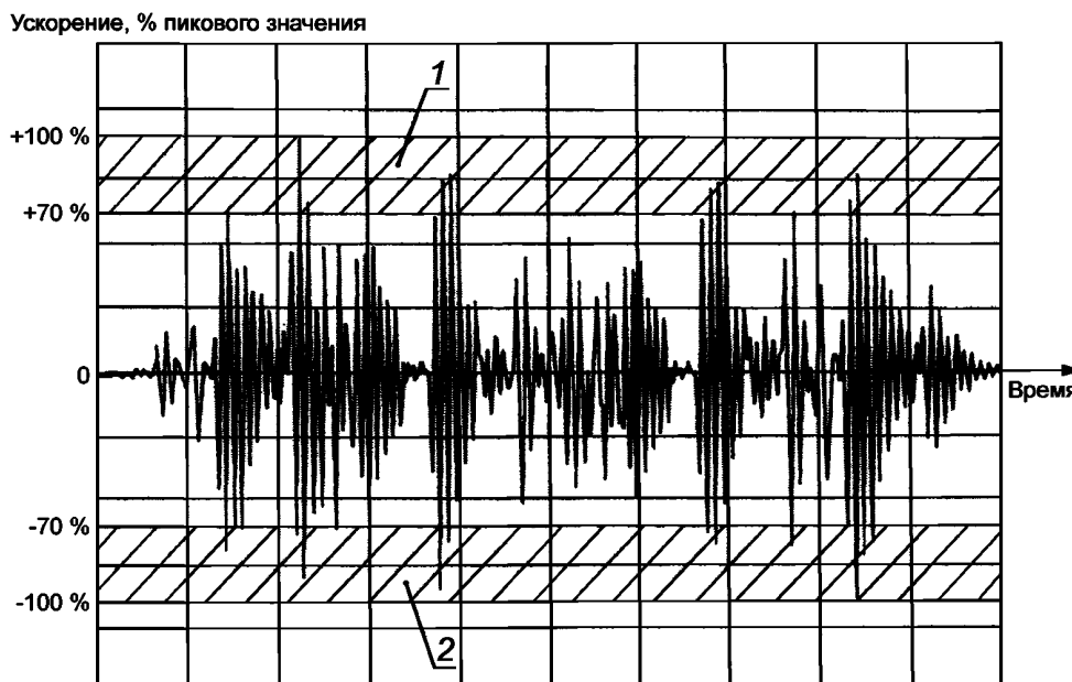
1 — область положительных пиков, превышающих пороговое значение (+ 70 %); 2 — область отрицательных пиков, превышающих пороговое значение (-70 %)
