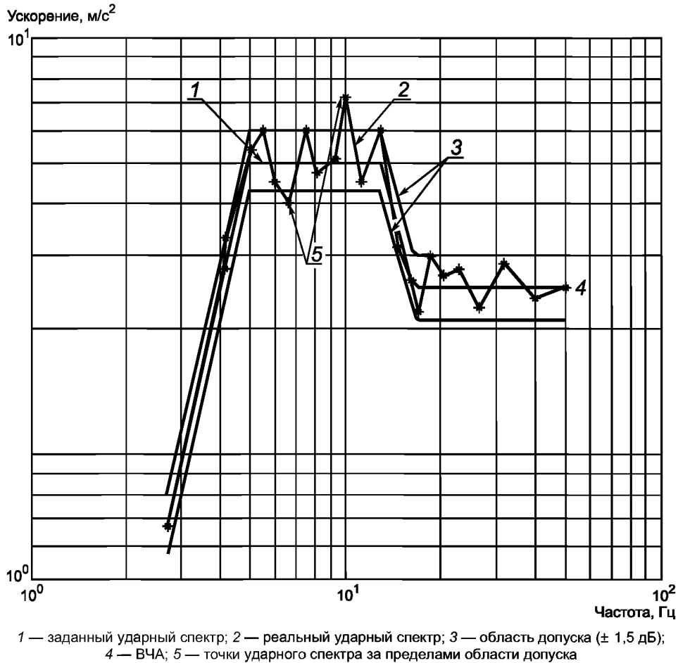
Рисунок 3 — Типичный график ударного спектра (в логарифмическом масштабе)
