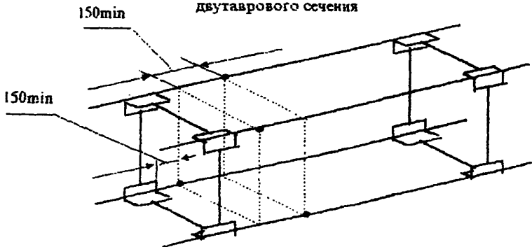
рисунк 2. Расположение сварных стыков в решетчатых металлоконструкциях
