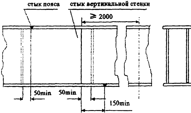
а) коробчатое сечение
