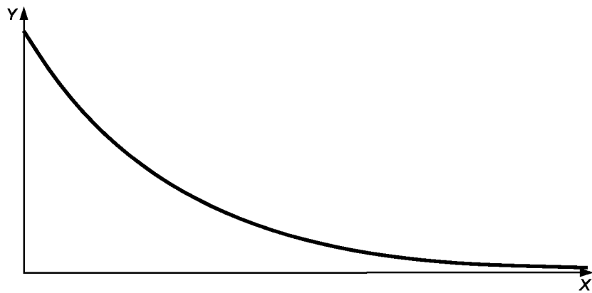
а) Плотность экспоненциального распределения
