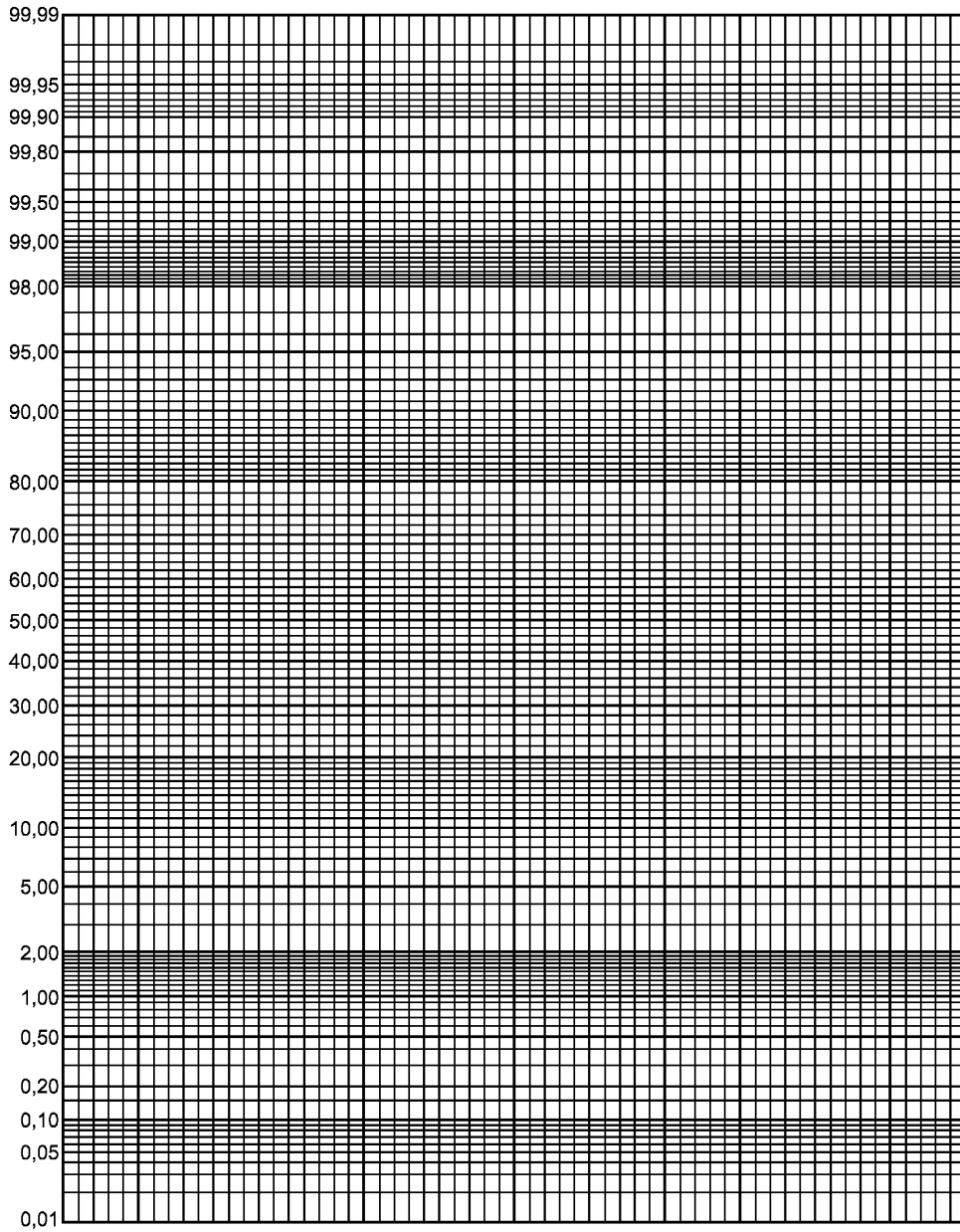
Рисунок А.1 — Вероятностная бумага для нормального распределения
