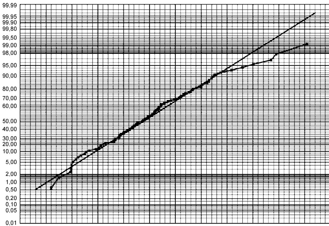
б) Функция распределения для случайной выборки объема 100 из логарифмически нормального распределения
