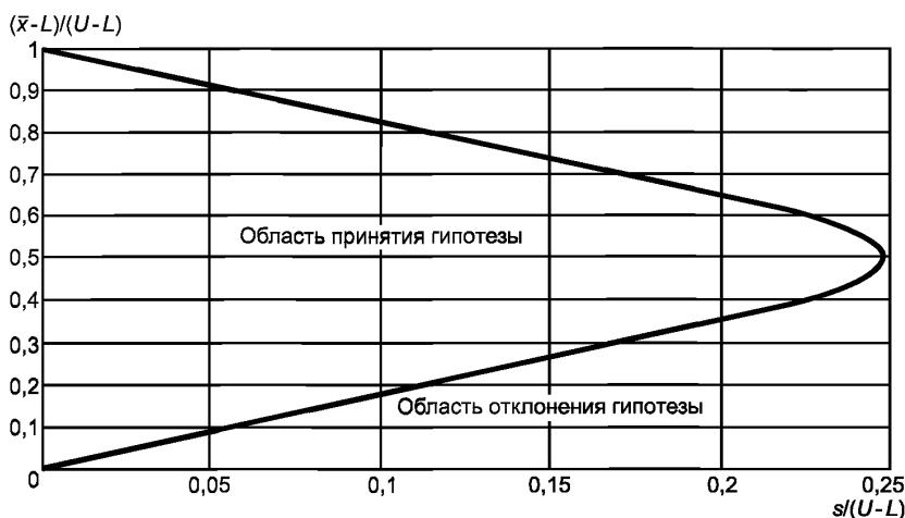
Рисунок 10 — Области принятия и отклонения гипотезы для объединенного контроля с двусторонними пределами поля допуска, s -метод, код объема выборки G, AQL = 1 %, n = 18 , p^* = 0,03323
