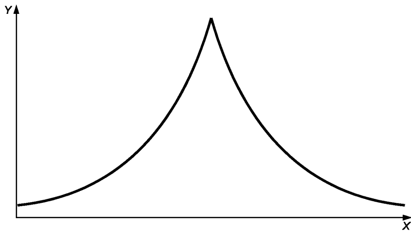
а) Плотность распределения Лапласа
