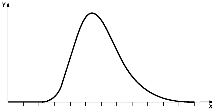
а) Плотность логарифмически нормального распределения
