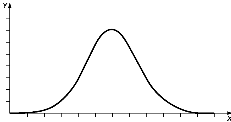
а) Плотность нормального распределения
