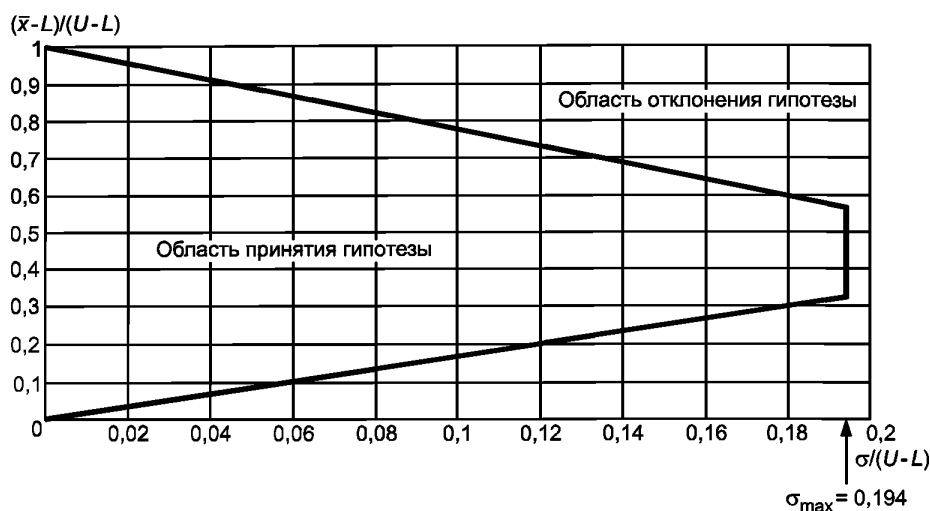
Рисунок 13 — Области принятия и отклонения гипотезы для сложного контроля двусторонних пределов поля допуска, \sigma -метод, код объема выборки М, объединенный AQL = 1,5 %, для верхнего предела AQL = 0,4 %
