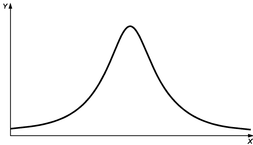
а) Плотность распределения Коши
