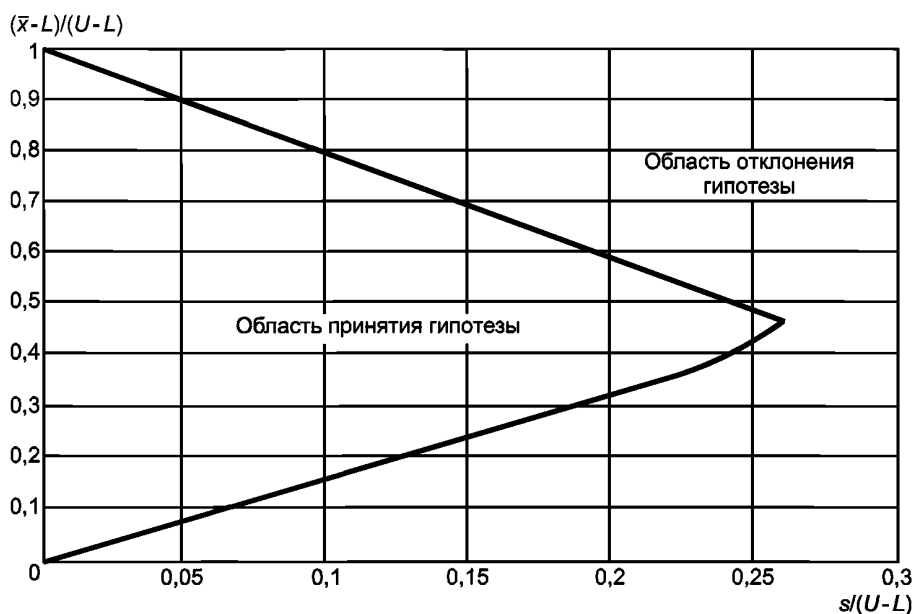
Рисунок 12 — Области принятия и отклонения гипотезы для сложного контроля двусторонних пределов поля допуска, s-метод, код объема выборки G, объединенный AQL = 1,5 %, для верхнего предела AQL = 0,4 %, n = 10 , p^* = 0,03323
