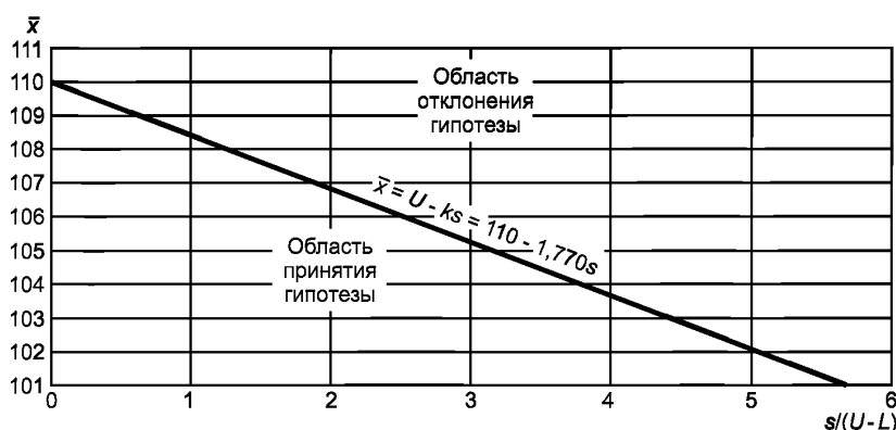
Рисунок 8 — Области принятия и отклонения гипотезы для единственного верхнего предела поля допуска 110, код объема выборки G, s -метод, AQL = 1 %, n = 18 , k = 1,770
