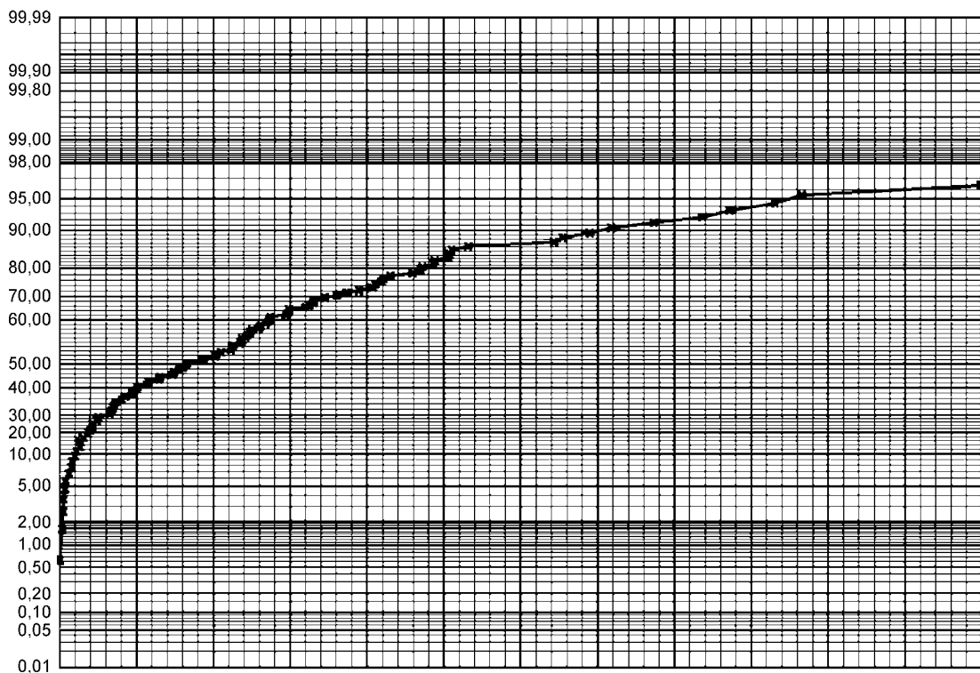
б) Функция распределения для случайной выборки объема 100 экспоненциального распределения
