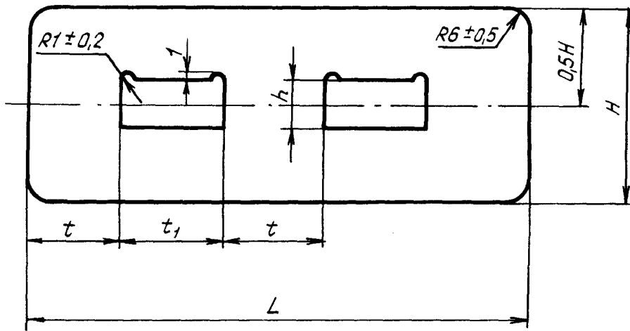
Развертка
