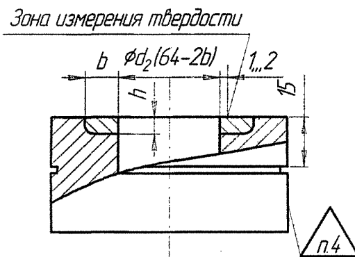
Рисунок Д.2 – Образец для замера твердости
