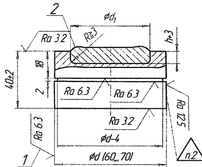
Рисунок Е.1 – Наплавленная заготовка 1 – заготовка 2 – наплавленный металл
