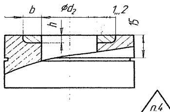
Рисунок Е.2 – Образец для замера твердости
