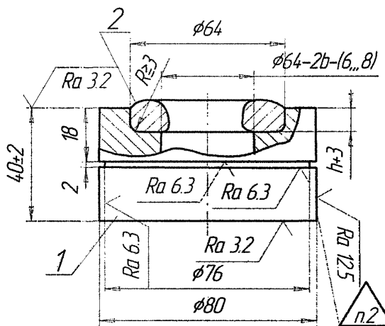
Рисунок Д.1 – Наплавленная заготовка
