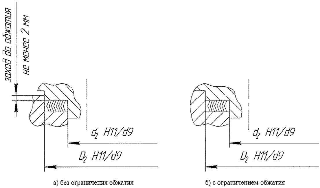
Рисунок 4 Соединение «замок»
