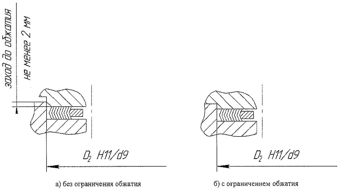
Рисунок 5 Соединение «выступ-впадина»
