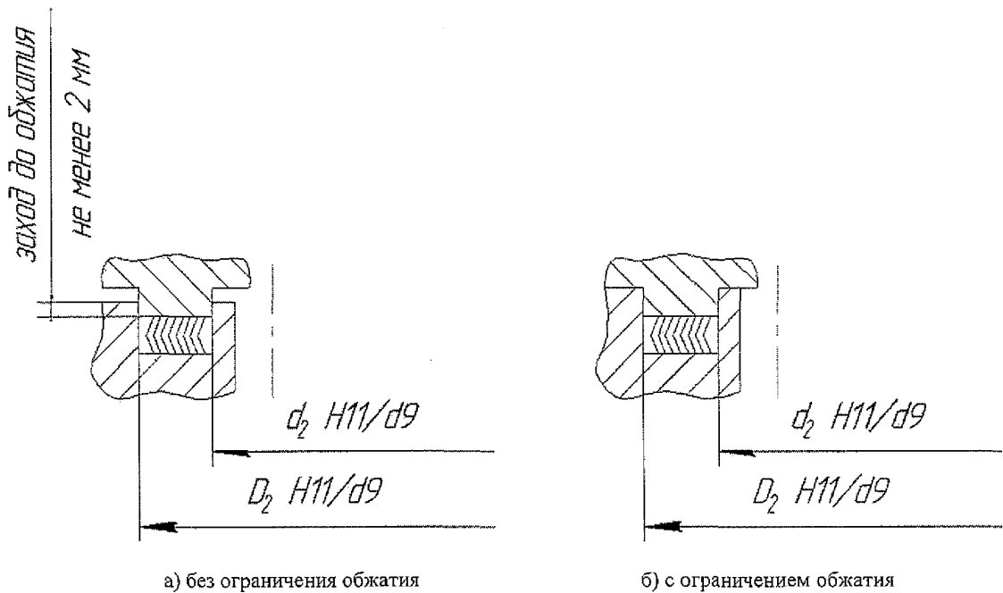
Рисунок 3 Соединение «шип-паз»
