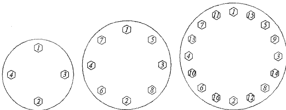
Рисунок 7 - Порядок затяжки болтов (шпилек) во фланцевом соединении
