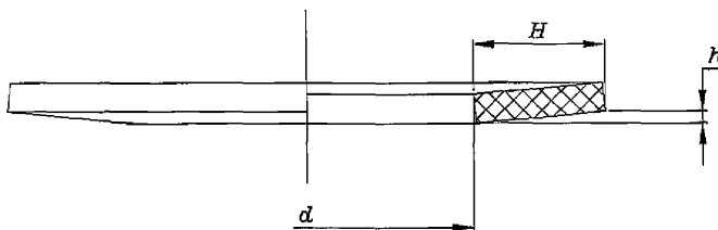
Рисунок 6 – Схема, характеризующая прогиб
