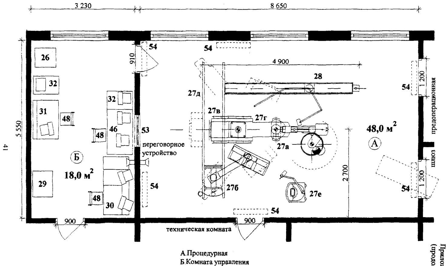
Рис. 3.6. Блок диагностики заболеваний сердца и сосудов
