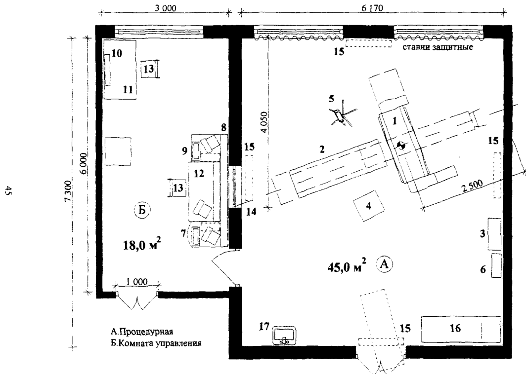
Рис. 4.1. Кабинет рентгенодиагностики методом рентгенографии и/или томографии
