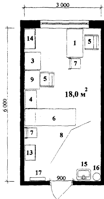
Рис 1.1. Кабинет исследований нарушений регионарного кровообращения
