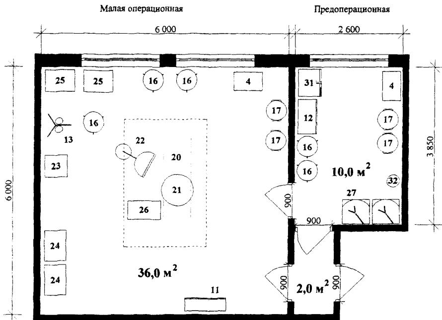
Рис .2.2. Эндоскопическая операционная
