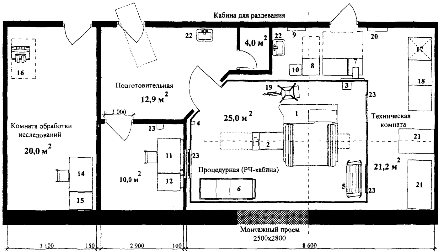
Рис. 5.1. Примерная габаритная схема кабинета магнитно-резонансной томографии
