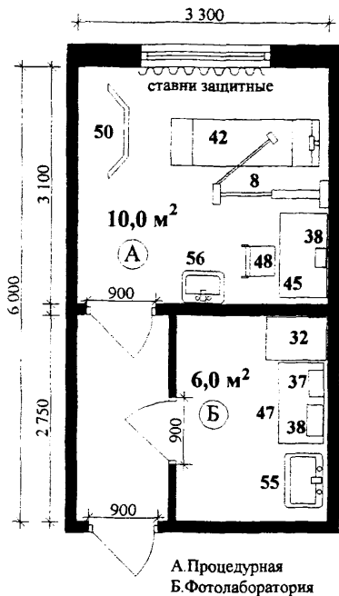
Рис.3.4. Кабинет рентгенодиагностики заболеваний зубов методом рентгенографии с дентальным аппаратом
