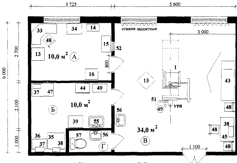
Рис. 3.1. Рентгенологический кабинет с универсальным рентгеновским аппаратом
