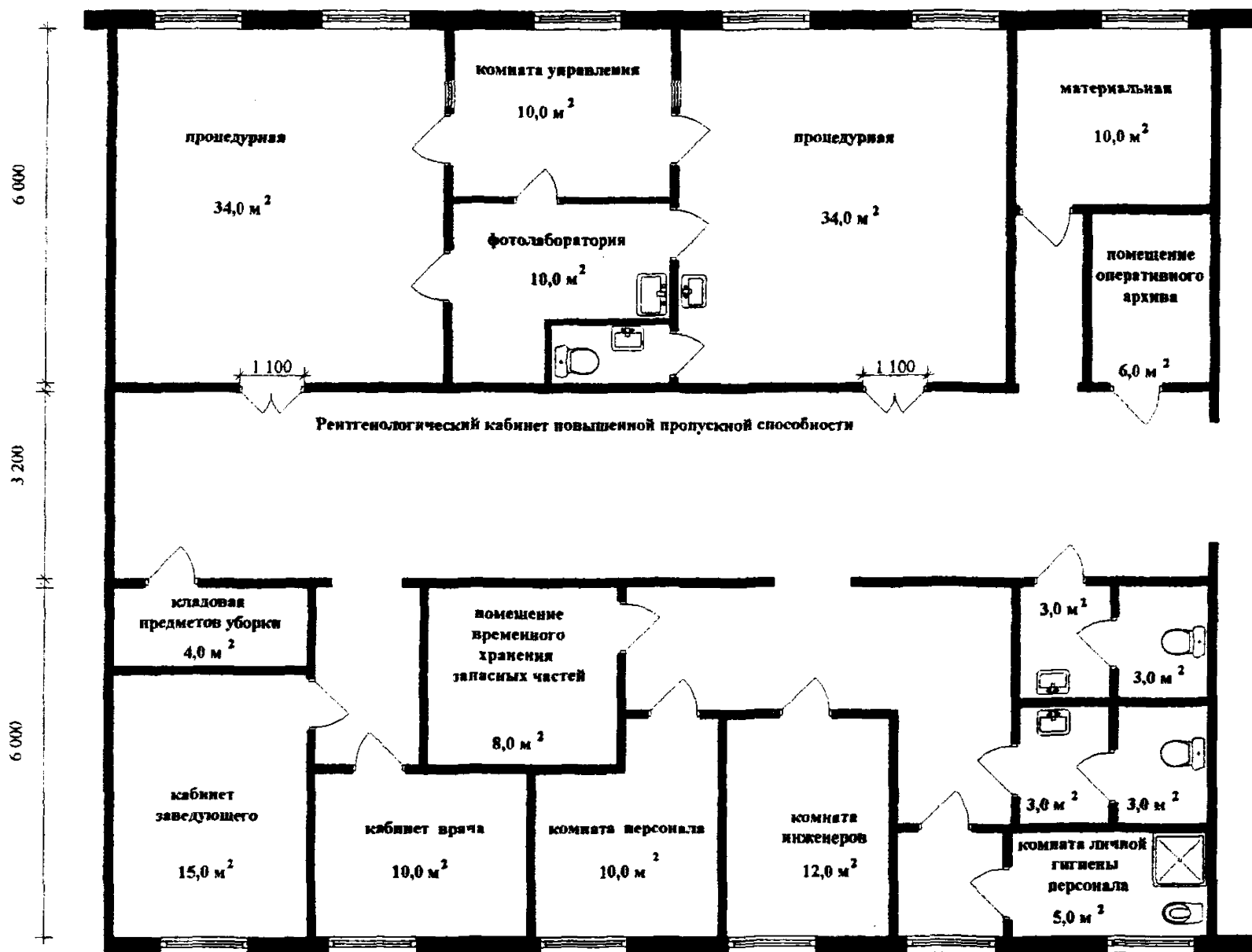
Рис.3.7. Фрагмент планировочного решения рентгенологического отделения
