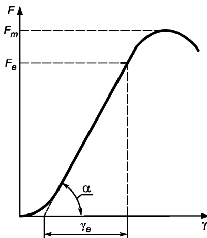
Рисунок 3 — Кривая зависимости сдвига от силы
