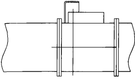
Вариант установки клапана КВП-Д в воздуховоде
