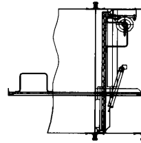
Вариант установки клапана КВП-Д стенового исполнения
