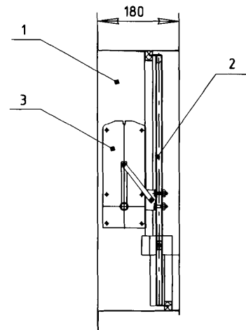
Схема конструкции клапана КВП-Д(С) с электромеханическим приводом
