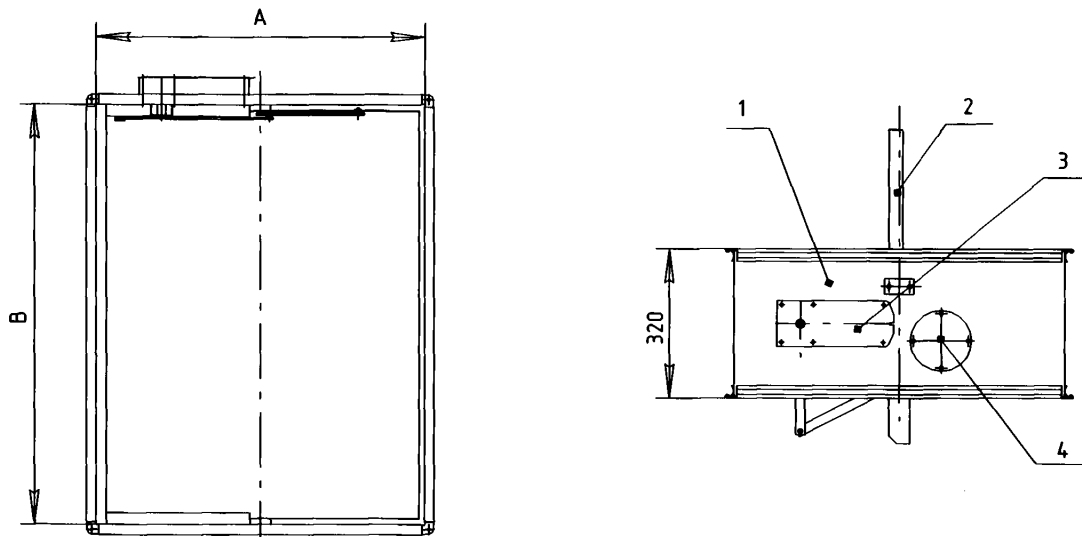
1 – корпус, 2 – заслонка, 3 – привод, 4 – смотровой лючок
