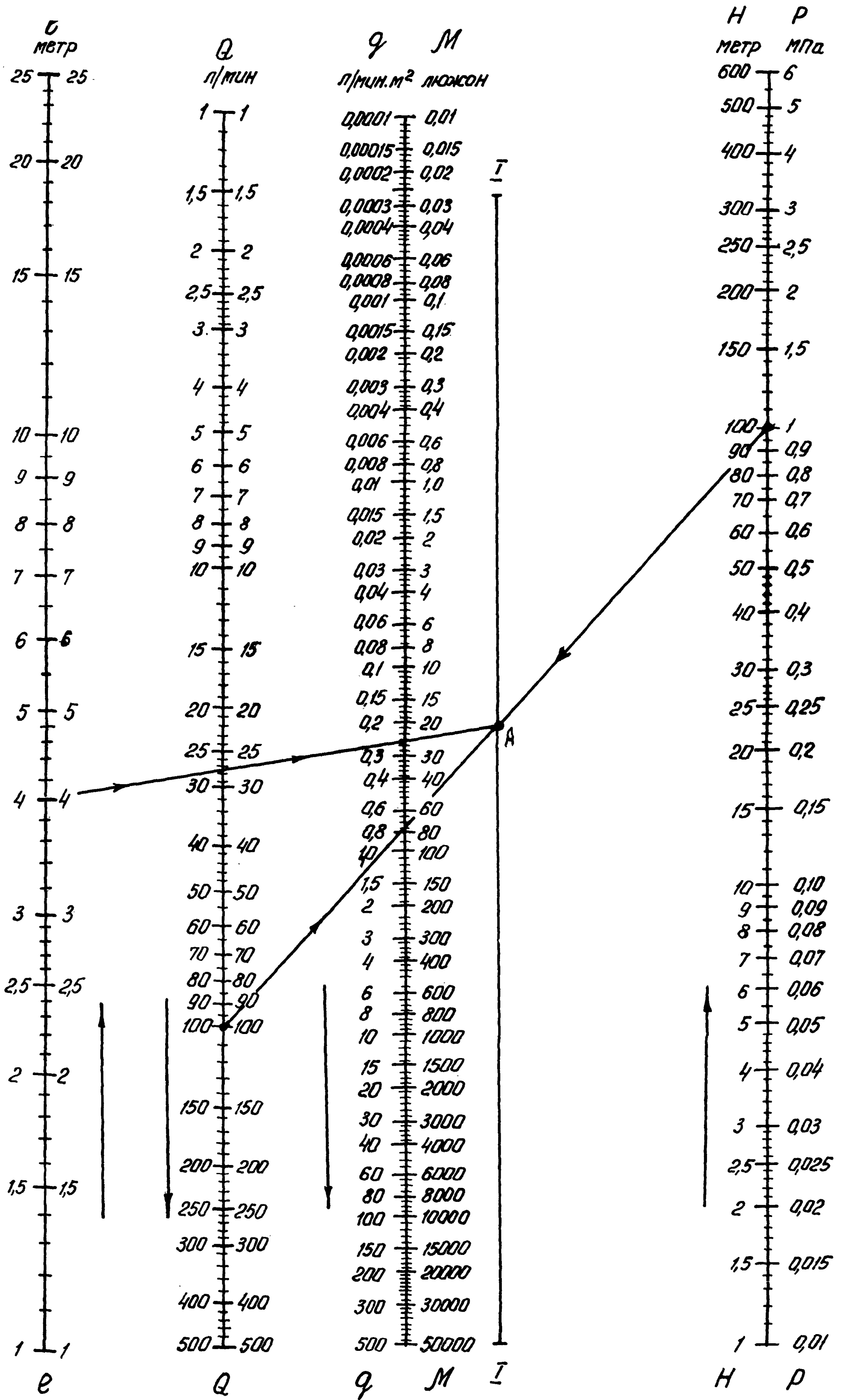
Рис. 2. Номограмма для определения удельного водопоглощения
