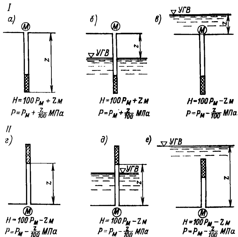
Рис. 1. Расчет действующего давления в зоне при гидравлическом опробовании
