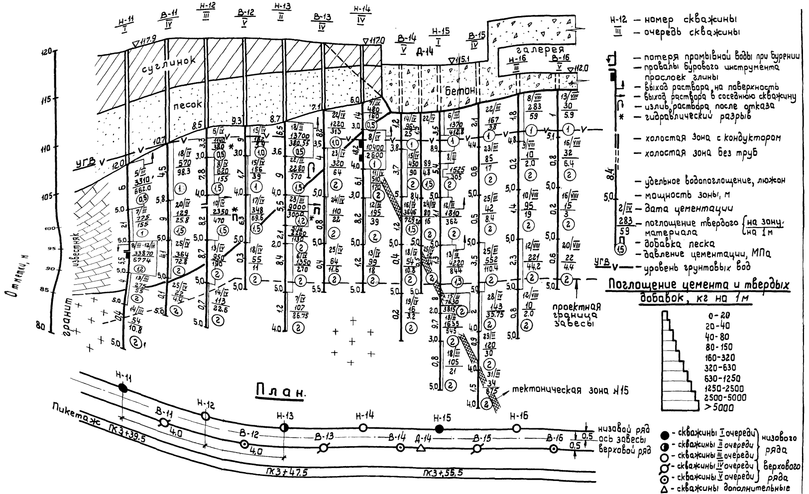
Исполнительный разрез по участку цементационной завесы. Масштаб 1:200.
