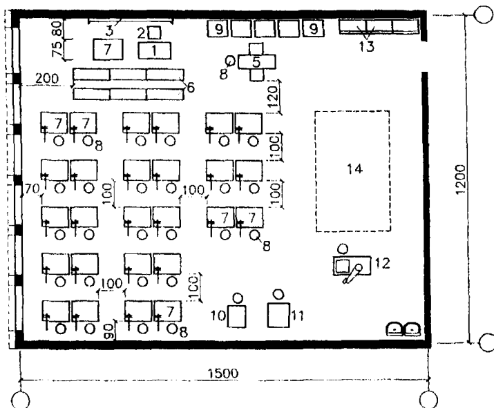
Рис.22. Пример планировки учебно-производственной слесарной (слесарно-сборочной) мастерской на 25 мест.
