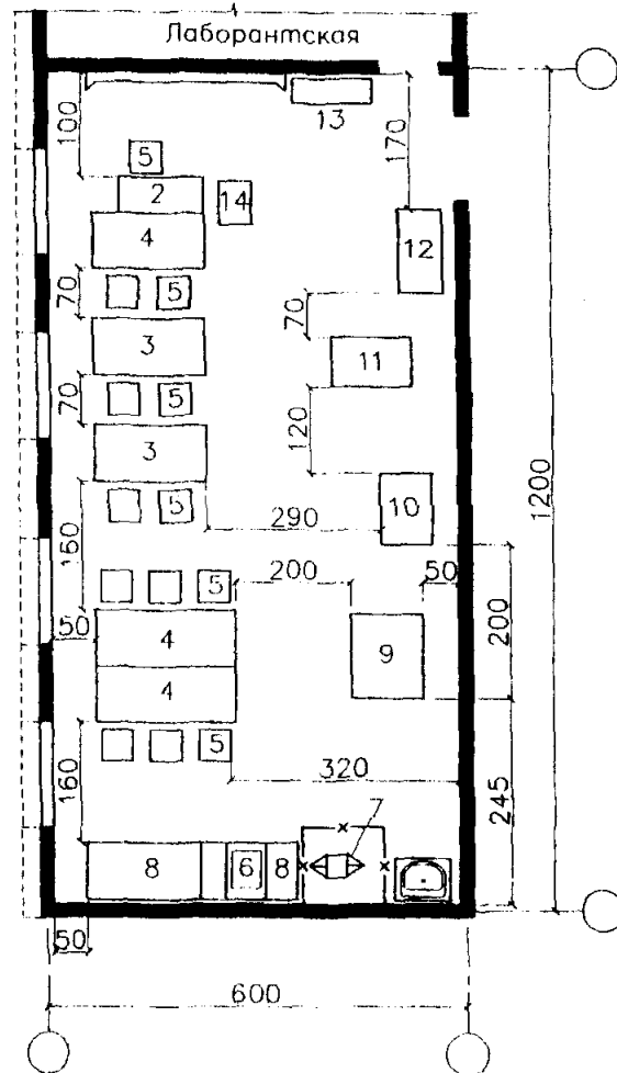
Рис.10. Пример планировки лаборатории материаловедения на13 мест.
