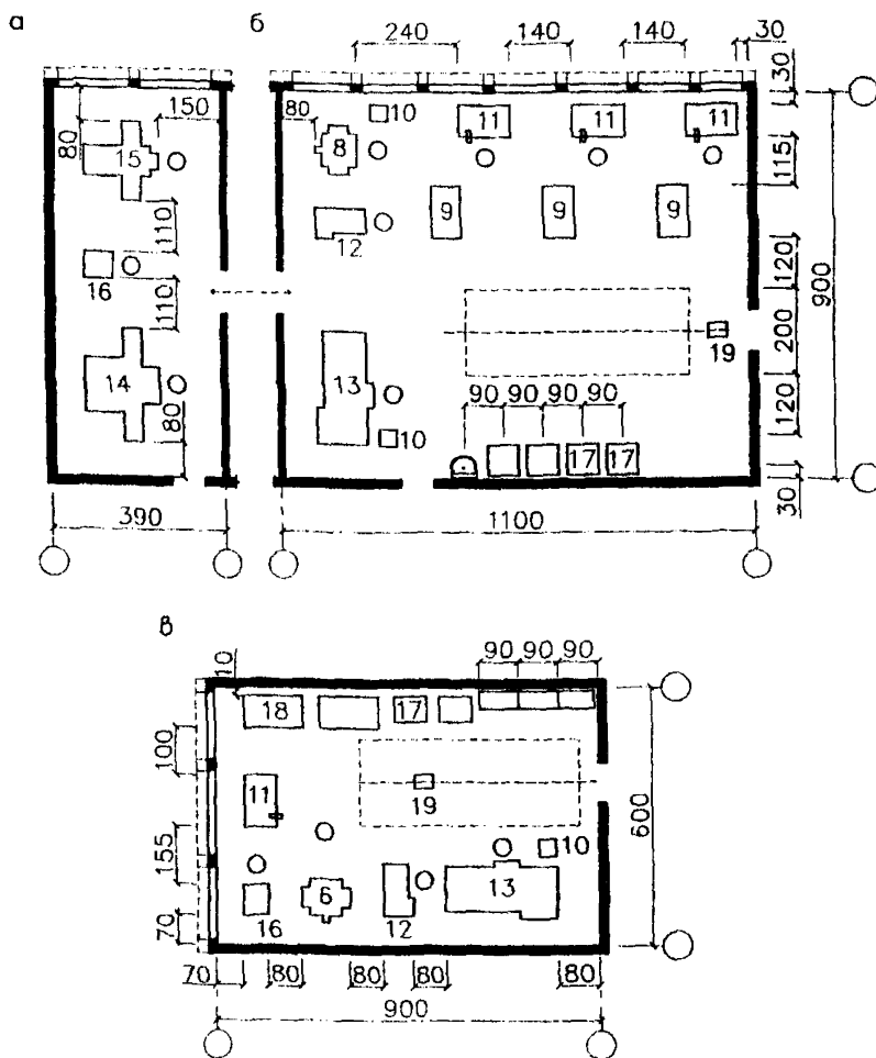
Рис.40. Примеры планировки производственно-вспомогательных помещений.
