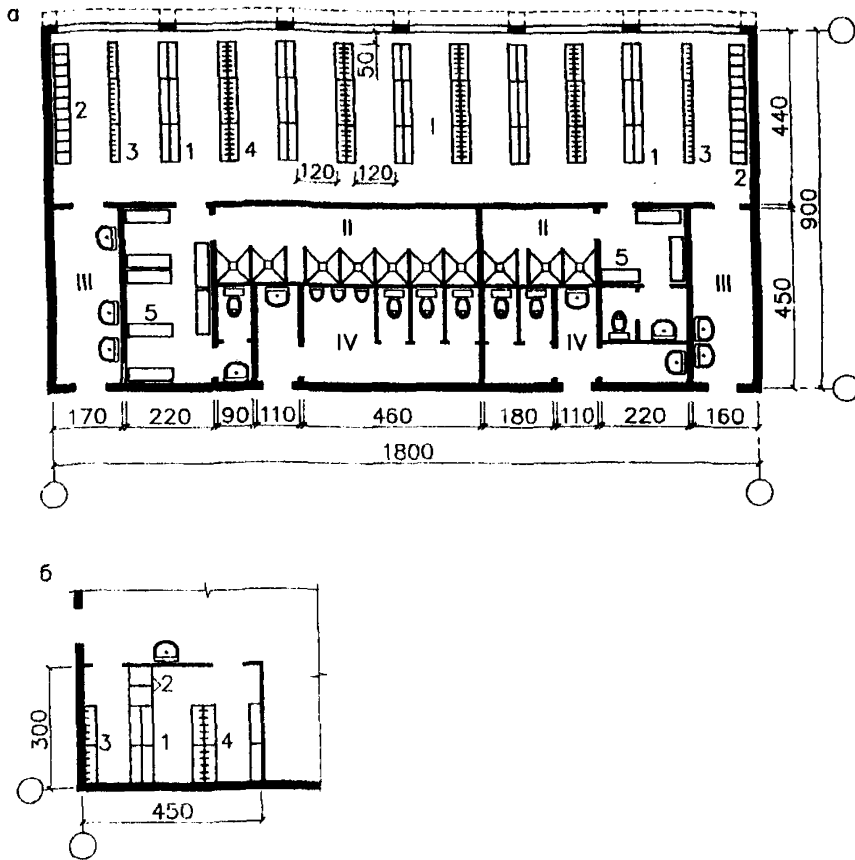
Рис.41. Примеры планировки санитарно-бытовых помещений. а - централизованный блок санитарно-бытовых помещений на 150 мест; б - гардеробная при механической мастерской.
