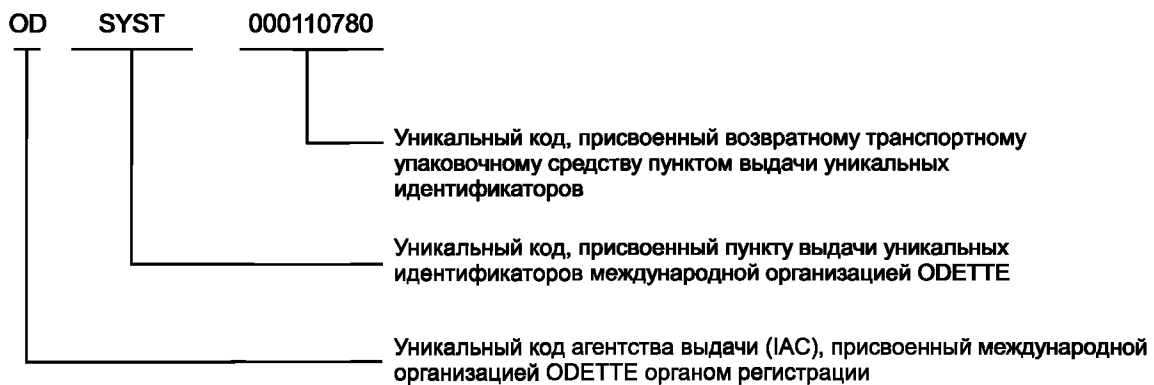
Рисунок А.2 — Уникальный идентификатор ODETTE для идентификации возвратных транспортных упаковочных средств
