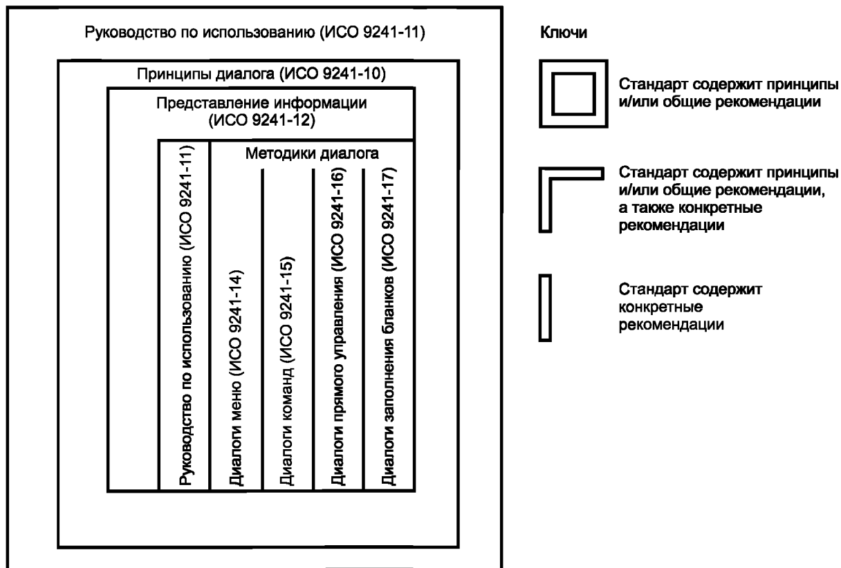
Рисунок А.1 — Соотношение частей программного обеспечения ИСО 9241
