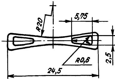
Развертка звена исполнения 1
