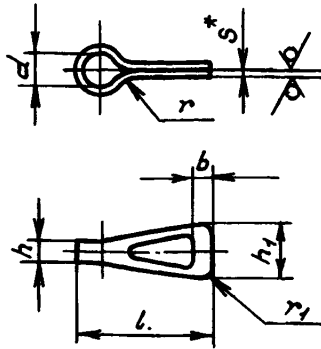
Развертка звена исполнения 1
