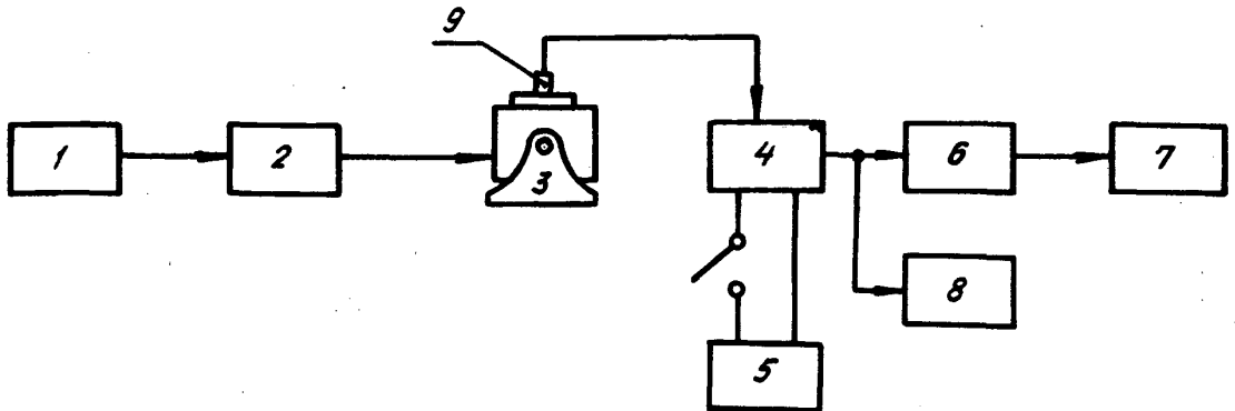
1 - аппаратура управления; 2 - усилитель мощности; 3 - вибратор; 4 - виброметр; 5 - фильтр; 6 - анализатор спектра; 7 - самописец уровня; 8 - осциллограф; 9 - виброизмерительный преобразователь
