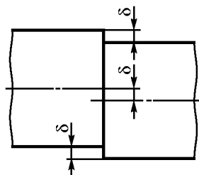
б — кольцевые сварные швы
