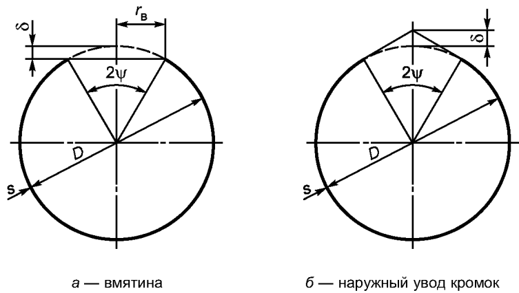
Рисунок А.4 — Локальная некруглость
