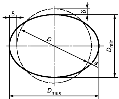
Рисунок А.3 — Общая некруглость
