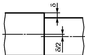
а — продольный сварной шов
