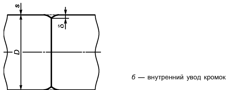
Рисунок А.2 — Увод кромок кольцевого шва
