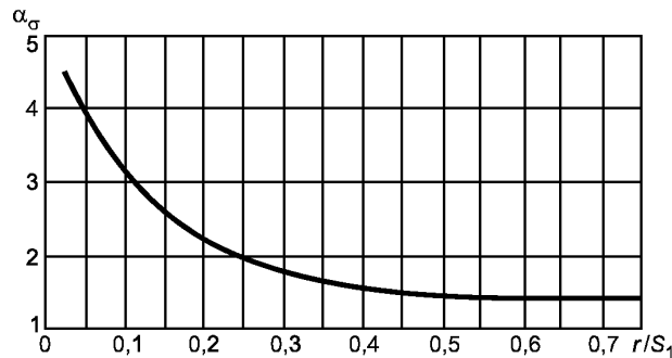
Рисунок 4 — График \alpha_\sigma
