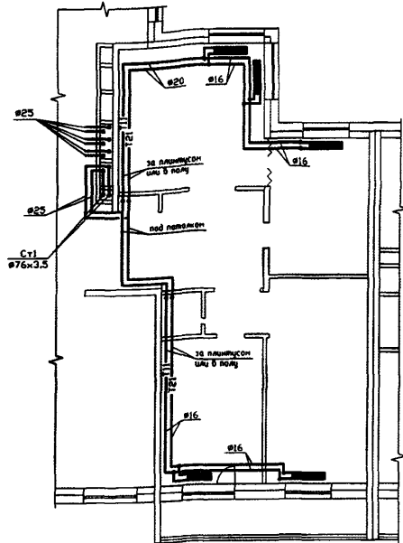
Рис. 2.5. Система отопления с плитусной разводкой теплопроводов по квартире
