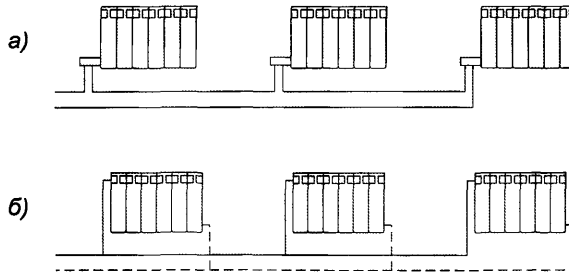
Рис. 2.3. Варианты присоединения секционных радиаторов «FARAL Green HP» и «FARAL Green» в горизонтальных системах отопления: а – однотрубной с одноузловым присоединением прибора; б – двухтрубной с разносторонним присоединением приборов
