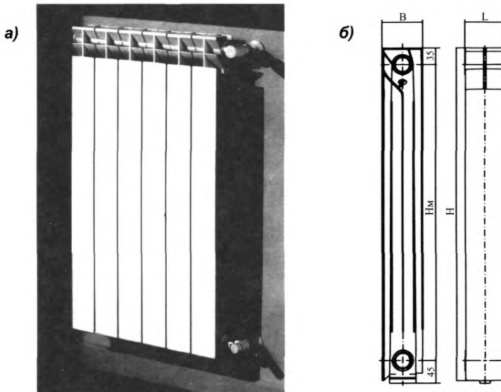
Рис. 1.1. Общий вид (а) и габаритные размеры (б) секции радиаторов «FARAL Green HP» и «FARAL Green»
