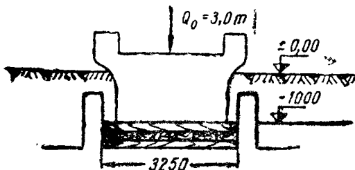
Рис. 5. Эскиз габаритов штамповочного молота (разрез)
