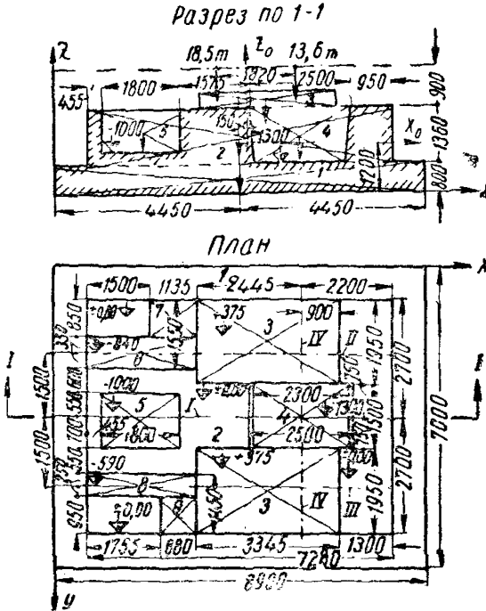
Рис. 4. Схема для вычисления центра тяжести фундамента и машины
