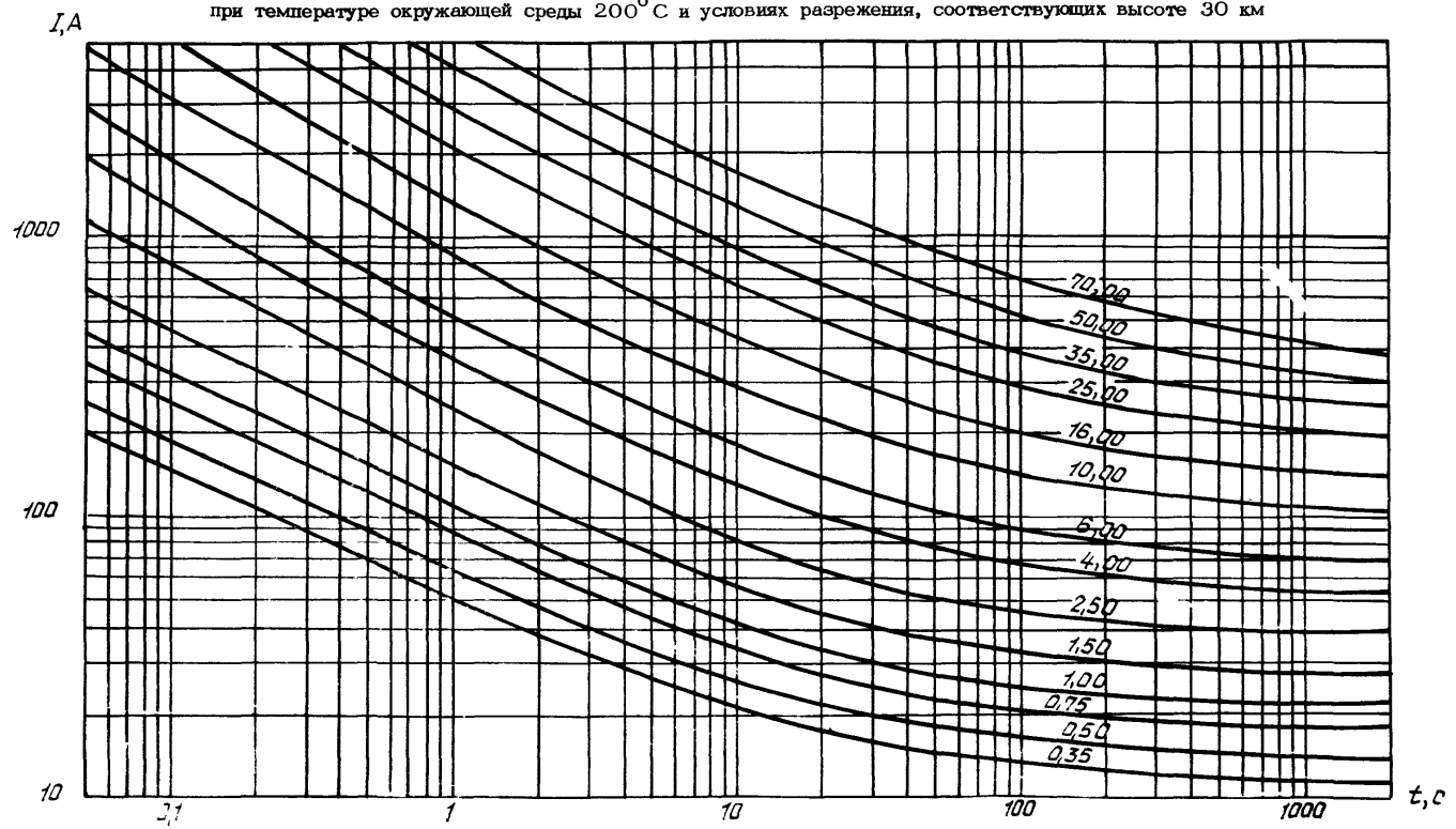
Цифры около кривых означают сечение провода в mm^2
