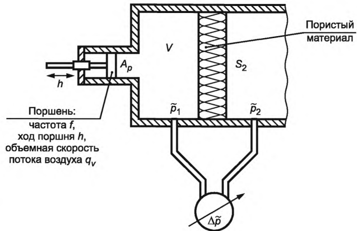
Рисунок 2 — Метод определения сопротивления продуванию переменным потоком воздуха (метод В) — основной принцип
