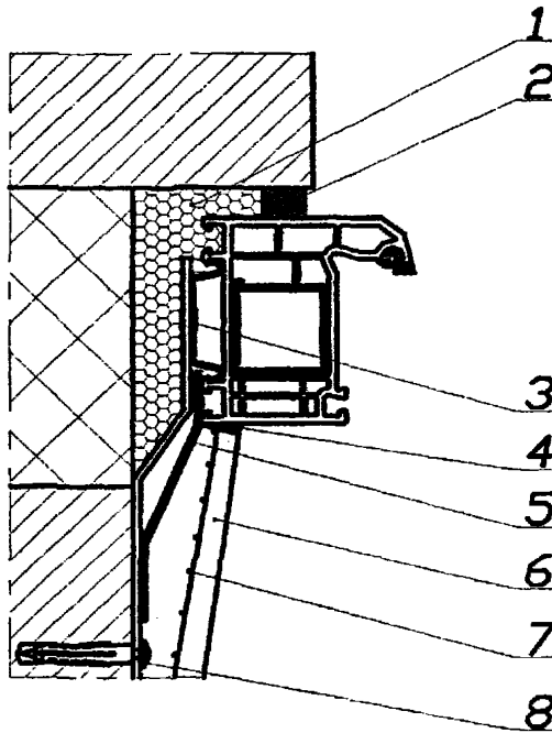
Рисунок 1 - Узел бокового примыкания оконного блока к проему с четвертью слоистой стены из кирпича с эффективным утеплителем и отделкой внутреннего откоса штукатурным раствором:
