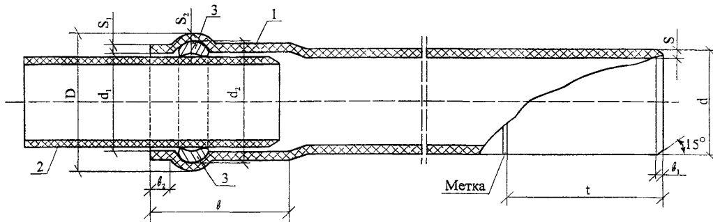
Рисунок 2 – Раструбное соединение напорных труб
