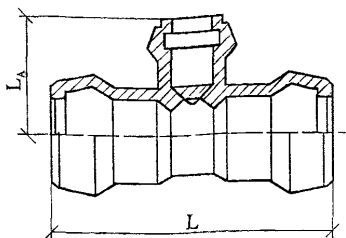
Рисунок 8 – Тройник с 2-я раструбами и фланец ММВ-КС
