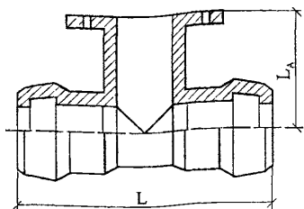
Рисунок 7 – Тройник с 2-я раструбами и фланец ММВ-КС
