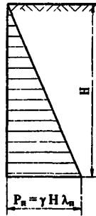
Рис. 10.10. Эпюра пассивного давления песка или супеси на стенку ограждения
