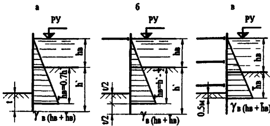
Рис. 17.2. СХЕМЫ ДЛЯ ОПРЕДЕЛЕНИЯ ГЛУБИНЫ ПРОНИКАНИЯ ВОДЫ МЕЖДУ ШПУНТОВОЙ СТЕНКОЙ И ВОДОНЕПРОНИЦАЕМЫМ ГРУНТОМ: а — при ограждениях, не имеющих распорных креплений; б — при ограждениях с одним ярусом крепления; в — при ограждениях с несколькими ярусами креплений
