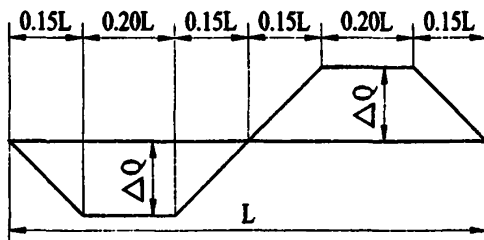
Рис. 23.2. Эюра поперечной силы \Delta Q от волновой нагрузки
