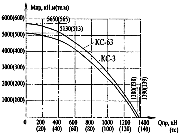
Рис.7.2. График предельных усилий на понтон при изгибе в плоскости бортов и при наличии местной нагрузки (гидростатического давления) W=18\text{кПа} ( 1.8\text{тс}/\text{м}^2 )
