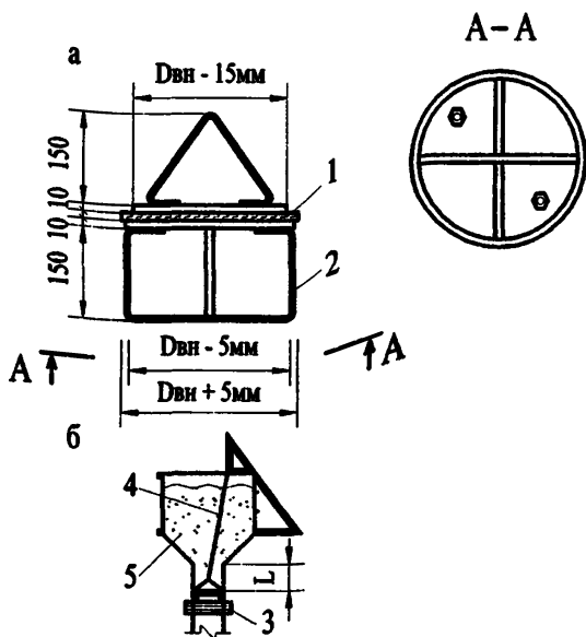
Рис. 24.2. СТАЛЬНАЯ ПРОБКА, УСТАНАВЛИВАЕМАЯ В ОСНОВАНИИ ВОРОНКИ ПРИ ПОДВОДНОЙ УКЛАДКЕ БЕТОНА В СКВАЖИНЫ
