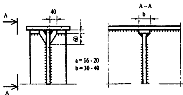
Рис. 11.1. ПРИМЫКАНИЕ РЕБЕР ЖЕСТКОСТИ К ПОЯСАМ БАЛКИ
