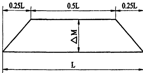
Рис. 23.1. Эюра момента \Delta M от волновой нагрузки
