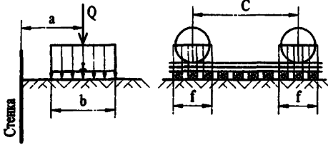
Рис. 10.3. К определению эквивалентной нагрузки от однорельсовой тележки на призме обрушения.
