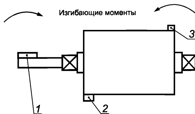
1 — полная шпонка; 2 — корректирующая масса 1; 3 — корректирующая масса 2
