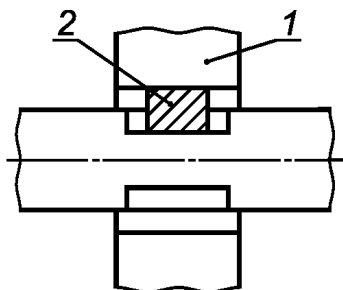
1 — насадка; 2 — шпонка половинной длины
