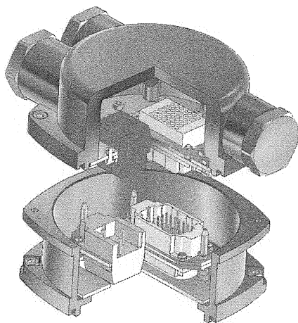
Рисунок Б.1 - Общий вид электрического разъема с расположением контактных групп
