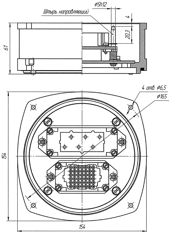
Рисунок А.5 - Габаритные и присоединительные размеры корпуса соединителя
