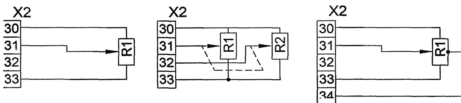
Рисунок Д.3 - Схема подключения резистивных датчиков
