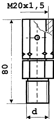
Соединение со стяжной муфтой для установки манометра на муфтовом клапане Рис.16
