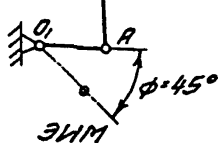
РИС.7. Сочленение ЭИМ с рычажным регулирующим клапаном (обратного типа, линейная характеристика сочленения):
