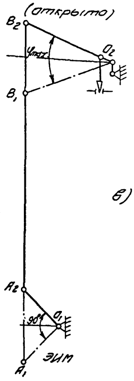
Рис. 6. Сочленение ЭИМ с рычажным регулирующим клапаном (прямого гмпа, линейная характеристика сочленения):
