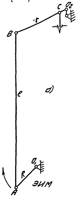
Рис. 6. Сочленение ЭИМ с рычажным регулирующим клапаном (прямого гмпа, линейная характеристика сочленения):
