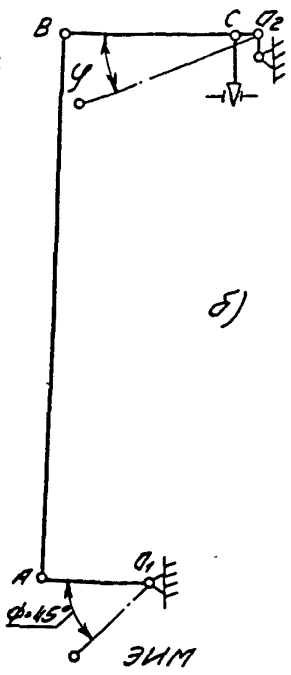
Рис. 6. Сочленение ЭИМ с рычажным регулирующим клапаном (прямого гмпа, линейная характеристика сочленения):
