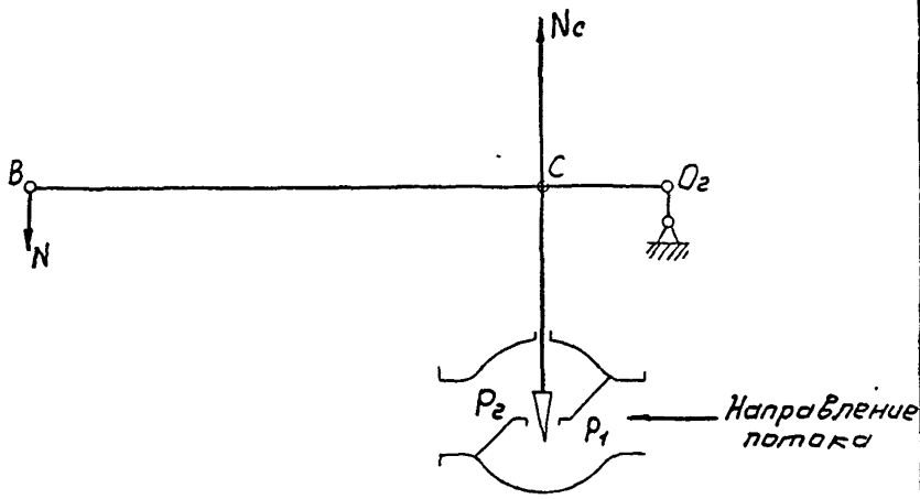
Рис. I. Односедельный регулирующий орган с рычажным приводом:
