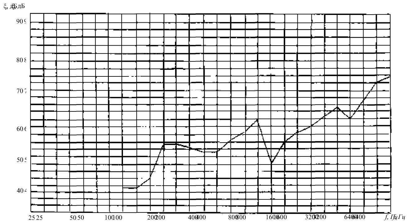
Рисунок А.1 Уровни вибрации маломощного переднего устройства усилителя гидравлическим сопротивлением
