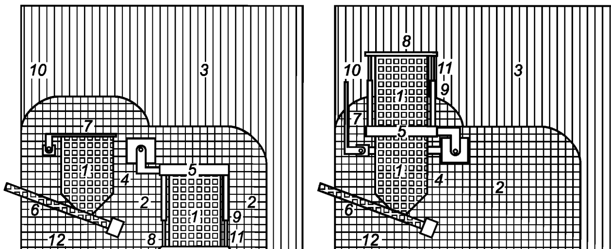
1 — зона класса 20; 2 — зона класса 21; 3 — зона класса 22; 4 — загрузочная воронка; 5 — мембранный клапан; 6 — винтовой конвейер; 7 — люк загрузочной воронки; 8 — барабанная платформа; 9 — гидравлические цилиндры; 10 — стена; 11 — барабан; 12 — основание
