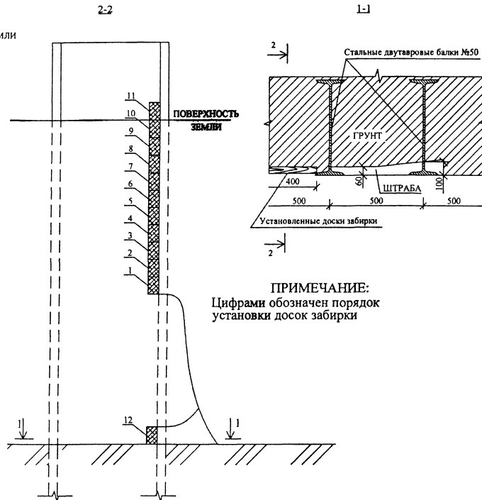
Рисунок 6 - Схема установки досок забирки
