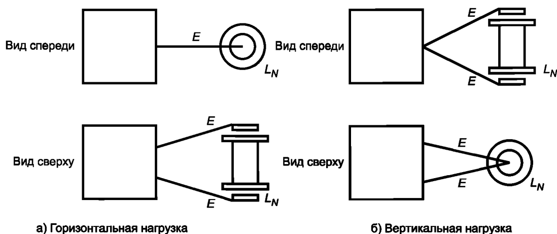
Рисунок 2 — Минимальные размеры металлической пластины заземления
