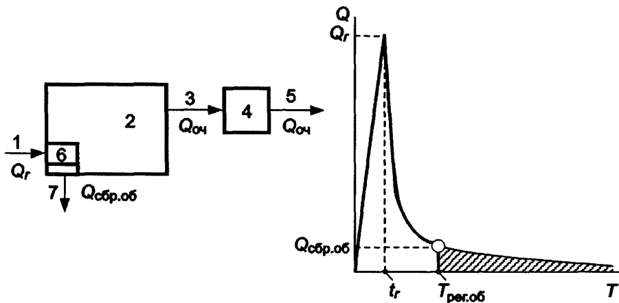
Рис. 1. Принципиальная схема регулирования дождевого стока перед очистными сооружениями и схематический расчетный гидрограф дождевого стока 1 – самотечный коллектор дождевой канализации; 2 – аккумулирующий (регулирующий) резервуар; 3 – трубопровод отведения стока на сооружения глубокой очистки; 4 – сооружения глубокой очистки; 5 – трубопровод отведения очищенного стока в водный объект или систему производственного водоснабжения; 6 – камера разделения стока по объему; 7 – сброс избыточного поверхностного стока в водный объект; □ часть объема дождя, поступающего в аккумулирующий резервуар для последующей очистки; ▨ часть объема дождя, отводимого в водный объект без очистки
