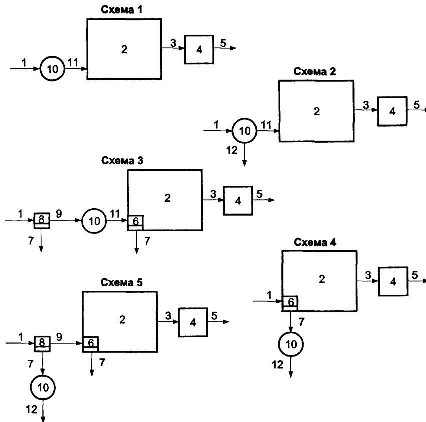
Рис. 2. Основные схемы перекачки дождевого стока
