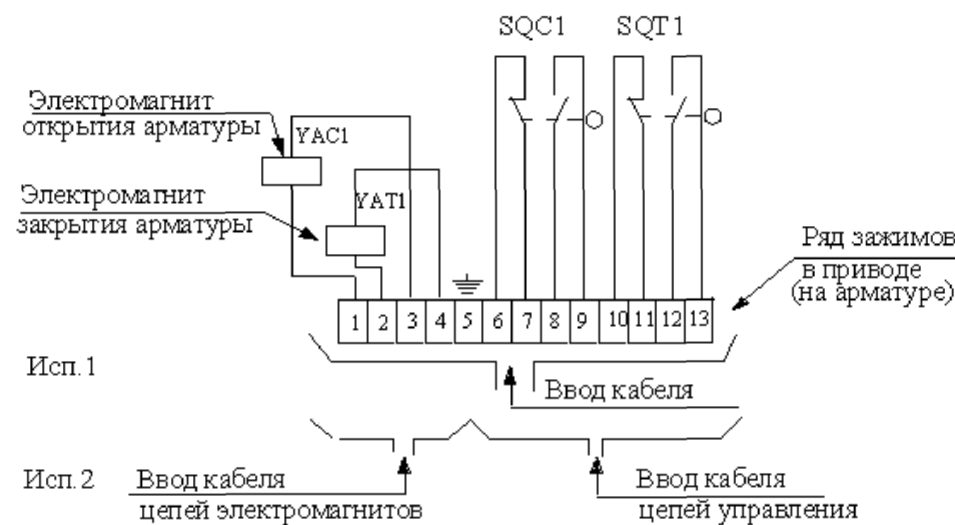
Рис. 4. Электрическая схема соединения электропривода запорно-регулирующей арматуры
