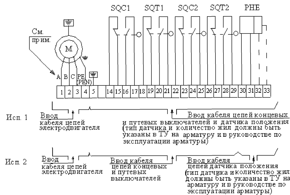
Рис. 2. Электрическая схема соединения электропривода запорной арматуры
