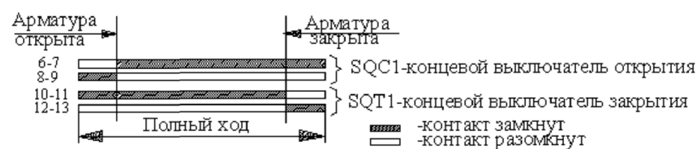
Рис. 5. Электрическая схема соединения электромагнитов управления и концевых выключателей отсечной пневмоприводной быстродействующей арматуры (нормально закрытой и нормально открытой) при установке под оболочкой и вне оболочки
