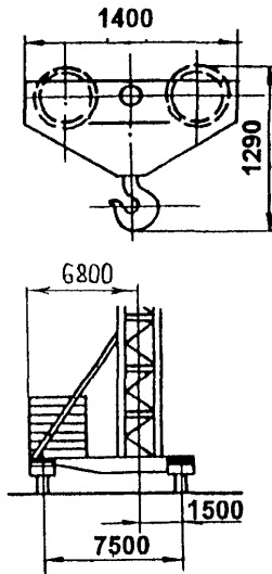
Крюковая подвеска
