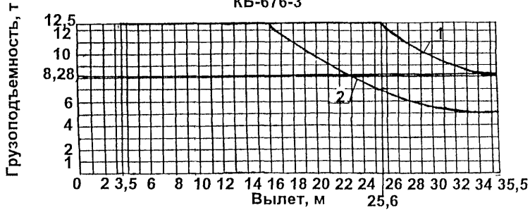
КБ-676-3
