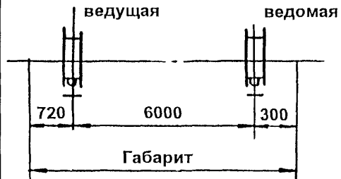
Тележки
