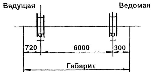
Тележки
