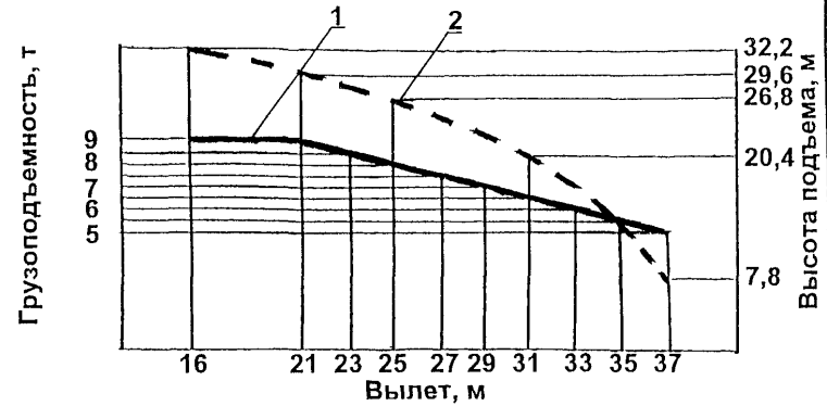
График грузоподъемности и высоты подъема
