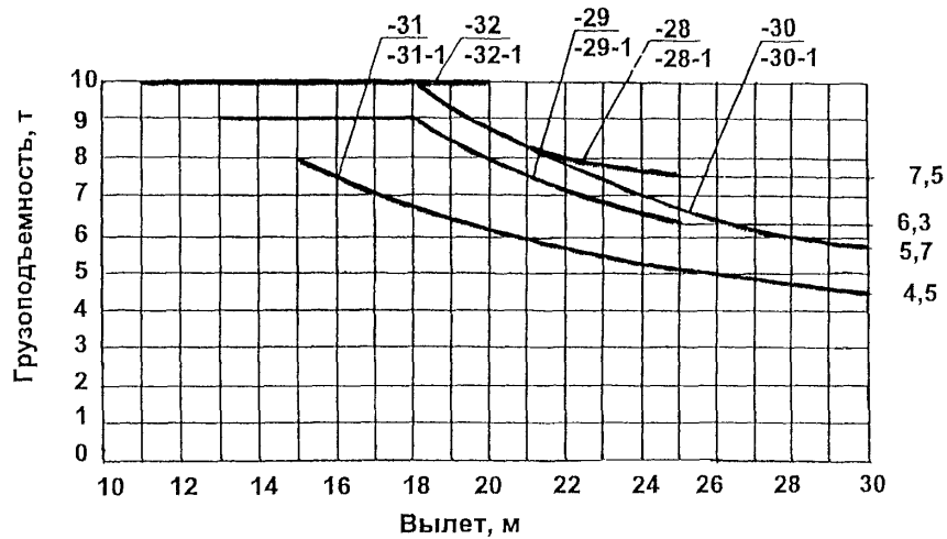
График грузоподъемности исполнений крана -28...32; -28-1...-32-1
