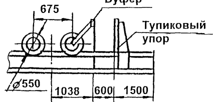
Буфер
