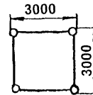
Наружные размеры стрелы с грузовой тележкой
