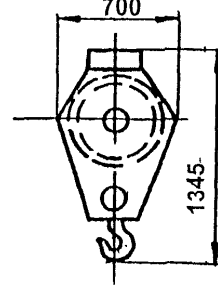
Крюковая подвеска
