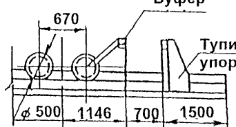
Буфер
