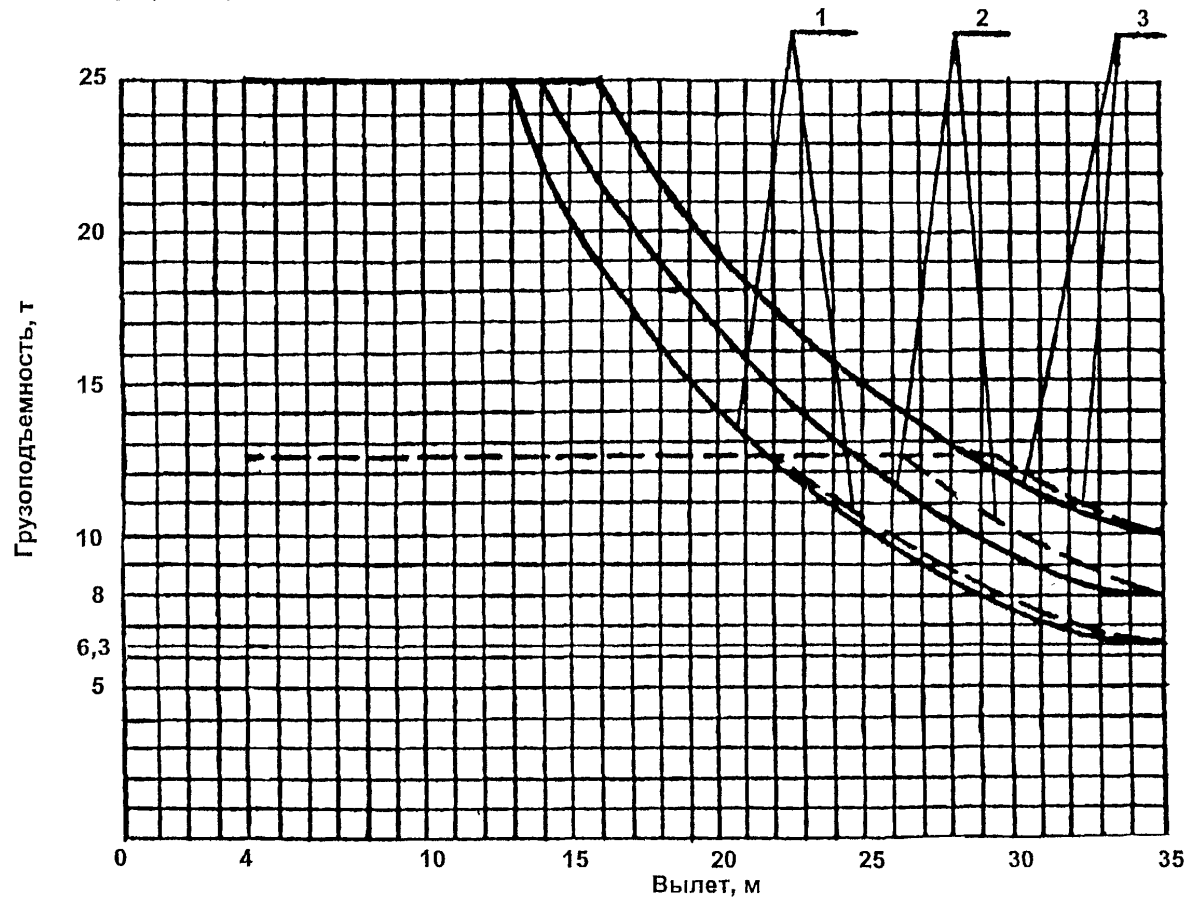
Графики грузоподъемности крана КБ-674А с улучшенной грузовой характеристикой
