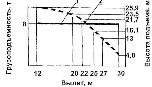
1 - график грузоподъемности 2 - график высоты подъема
