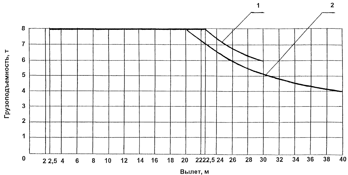
График грузоподъемности
