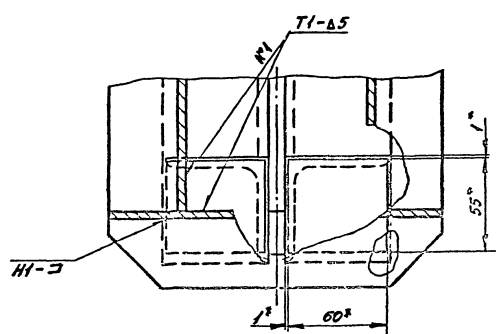
B-B M1:2
