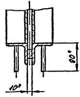
B-B M1:2
