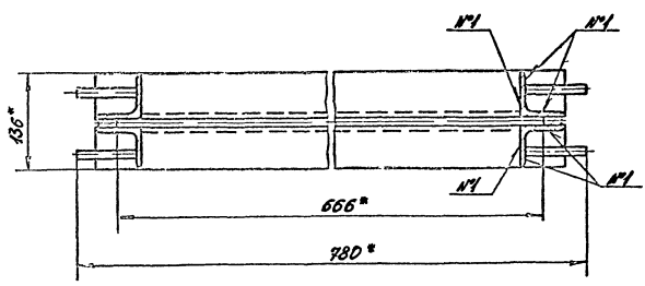
A-A M1:5
