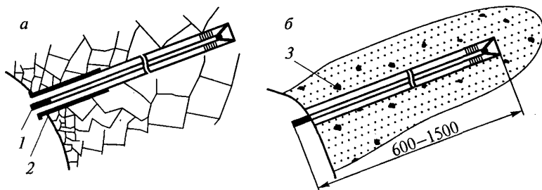
Рис. 4. Анкеры распорного типа для закрепления маркшейдерских пунктов:
