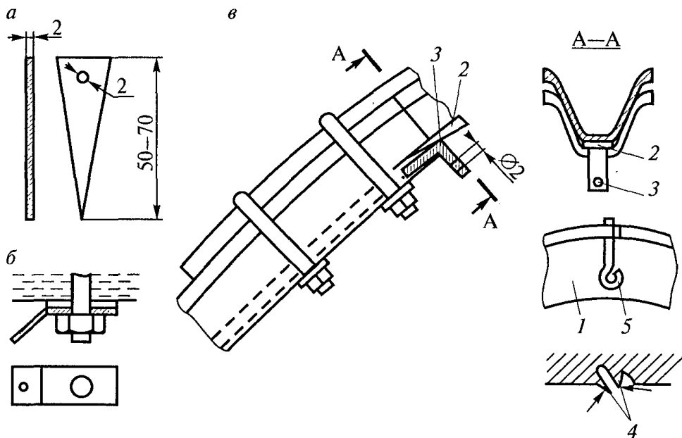
Рис. 5. Центры временных пунктов:
