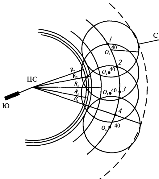
Рис. 6. Схема построения нормальных сечений по замораживающим скважинам
