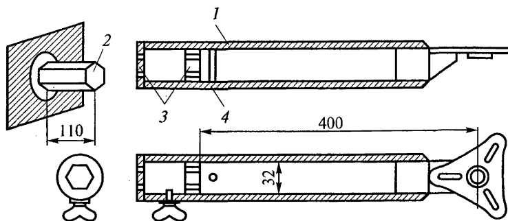
Рис. 3. Центр пункта в боках выработки
