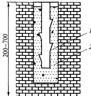
Рис. 1. Центр пункта (репер) в подошве выработки:
