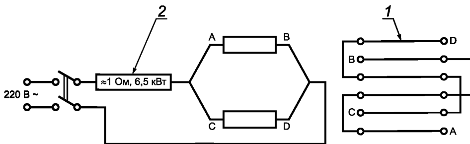
Рисунок 2 — Схема питания для нагревательных стержней
