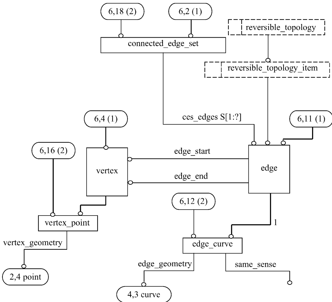
Рисунок С.6 — aic_edge_based_wireframe — EXPRESS-G диаграмма 6 из 6
