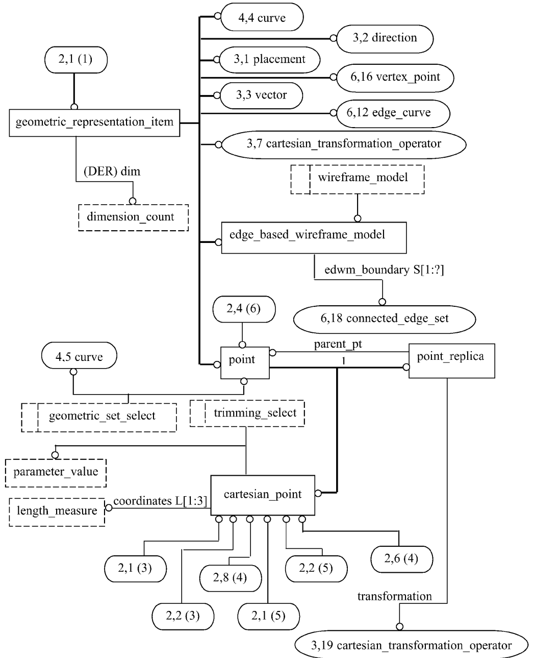
Рисунок С.2 — aic_edge_based_wireframe — EXPRESS-G диаграмма 2 из 6
