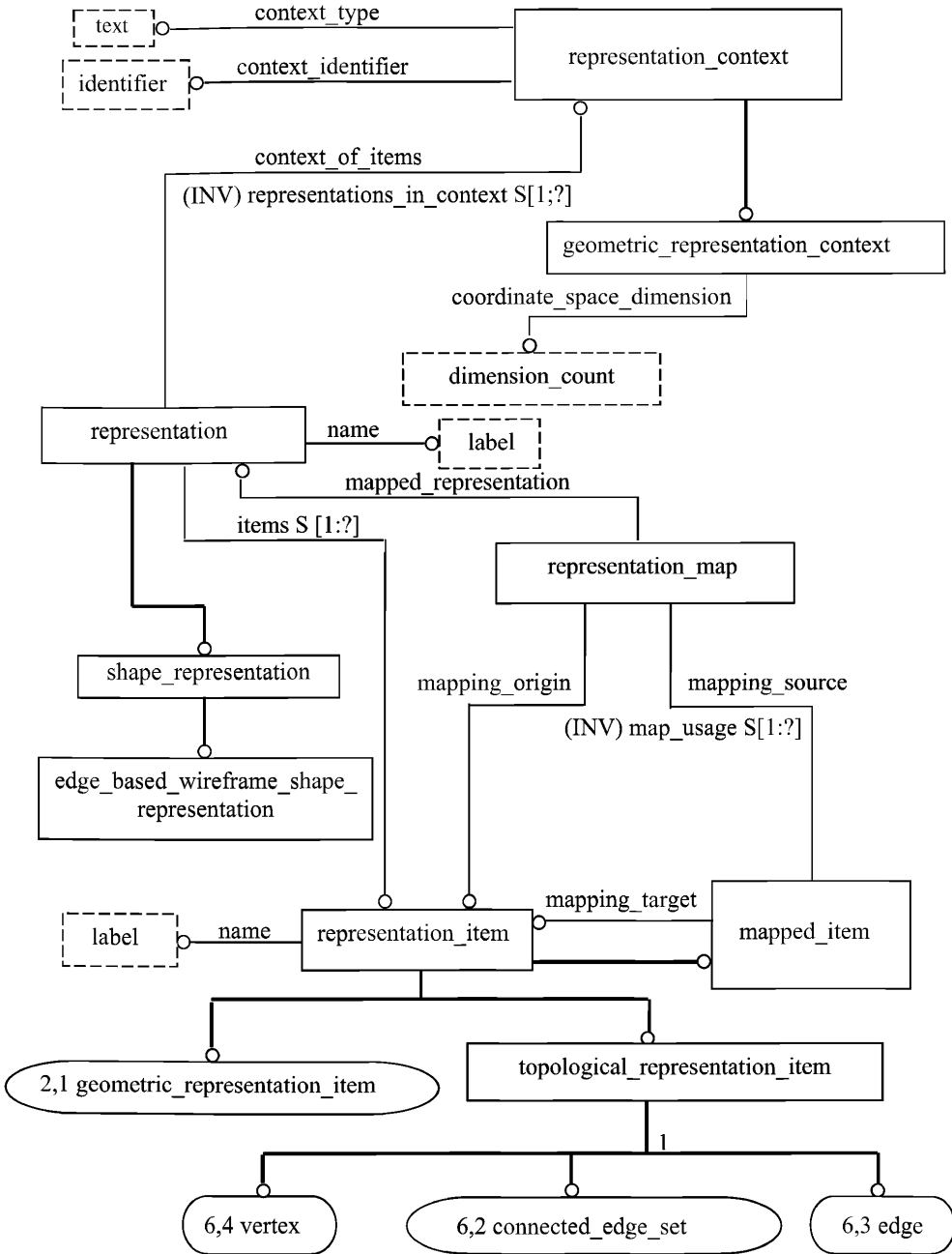
Рисунок С.1 — a1c_edge_based_wireframe — EXPRESS-G диаграмма 1 из 6
