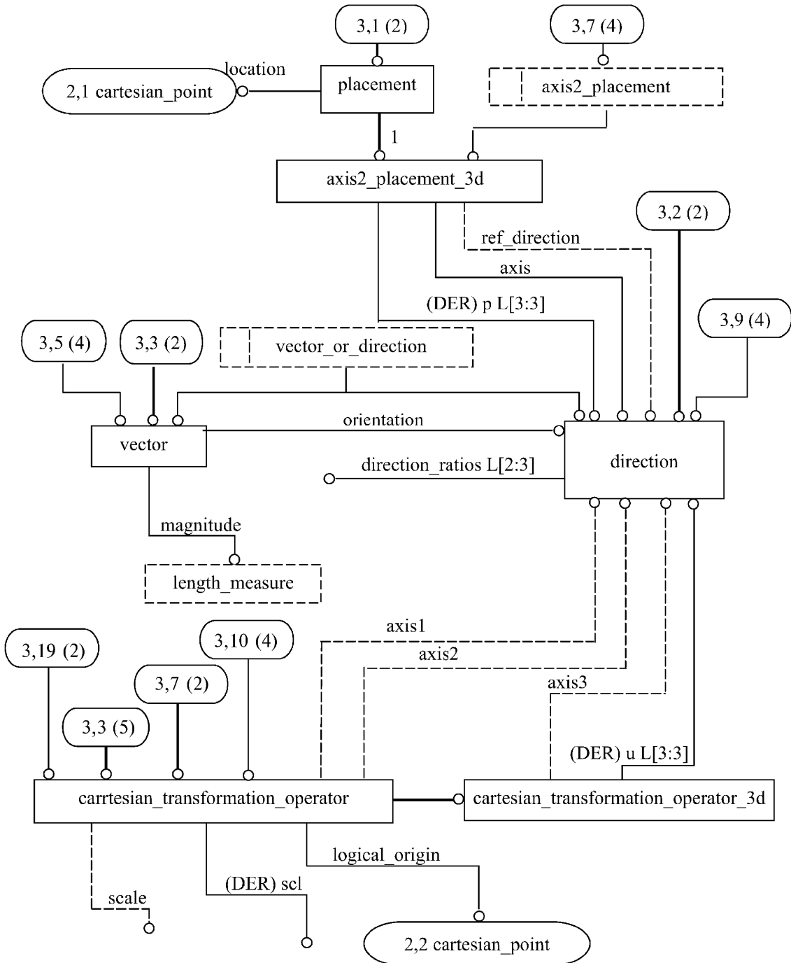
Рисунок С.3 — aic_edge_based_wireframe — EXPRESS-G диаграмма 3 из 6
