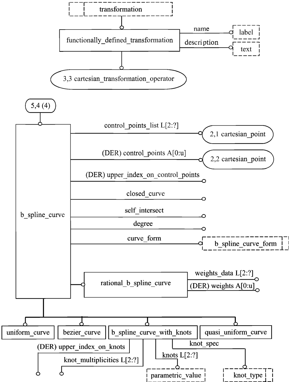
Рисунок С.5 — aic_edge_based_wireframe — EXPRESS-G диаграмма 5 из 6
