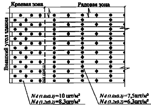
Фрагмент теплоизоляции стен выше отм. + 40,0 от уровня отмостки здания
