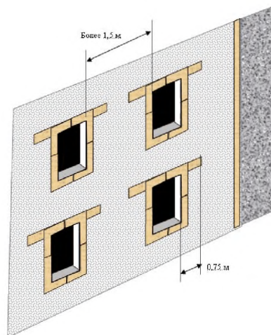
Схема 7.2 Размещение противопожарных расщечек вокруг проемов и в зоне примыкания.
