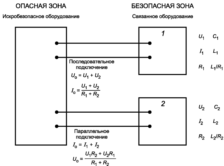
Рисунок В.3 — Произвольно подключенные источники питания
